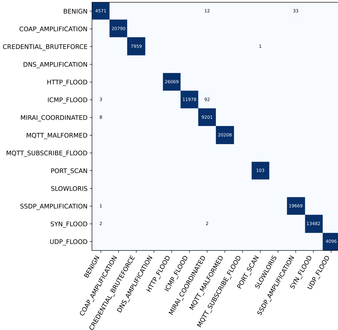
Matriz de confusión — mlp
