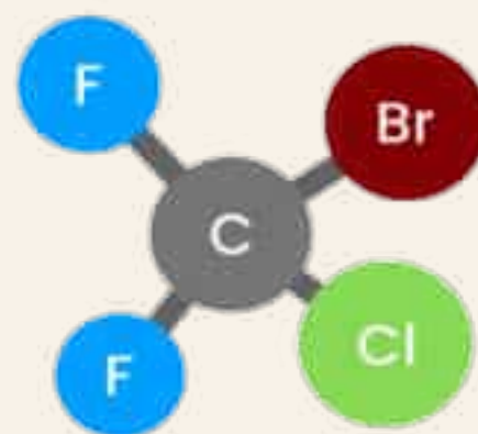
Halon 1211 \text{CF}_3\text{ClBr}
