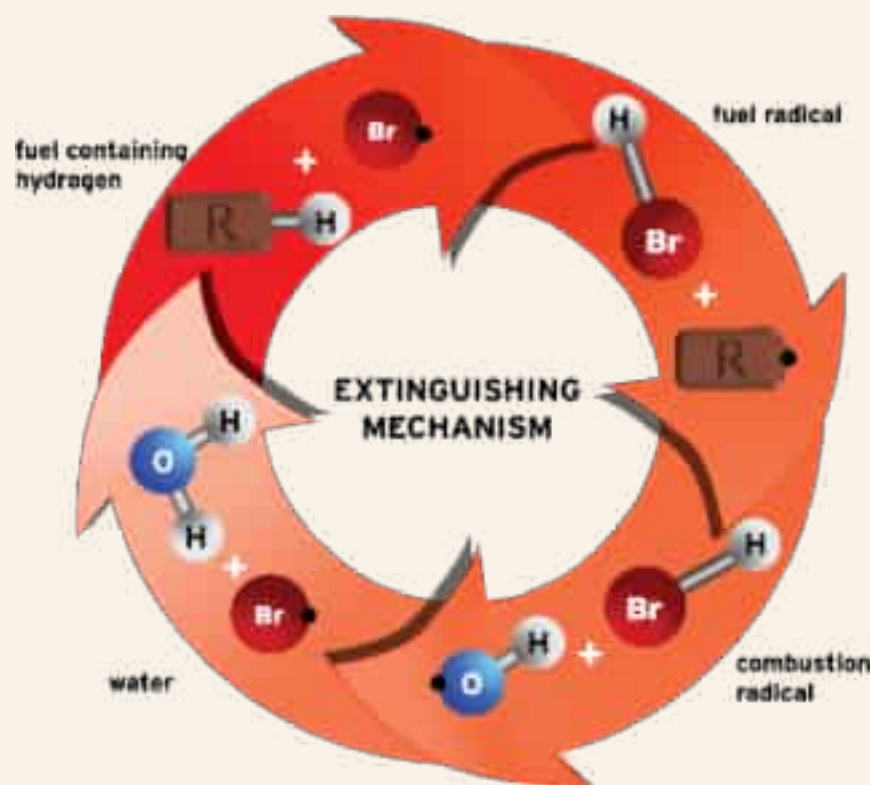
Halon 1211 \text{CF}_3\text{ClBr}
