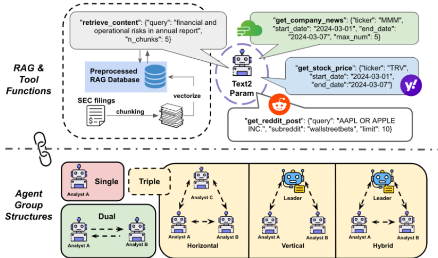
Hình 1: Khung làm việc hợp tác giữa các tác tử, tích hợp RAG và chức năng gọi công cụ một cách thống nhất.
