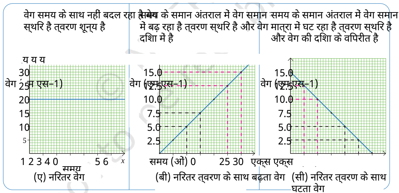
चित्र 4.17: चलती कार का वेग-समय ग्राफ
