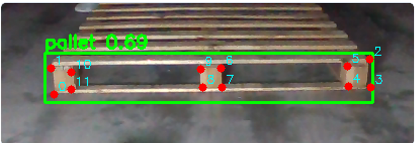
파렛트 키포인트 라벨링 예시 (인덱스 0~11)
