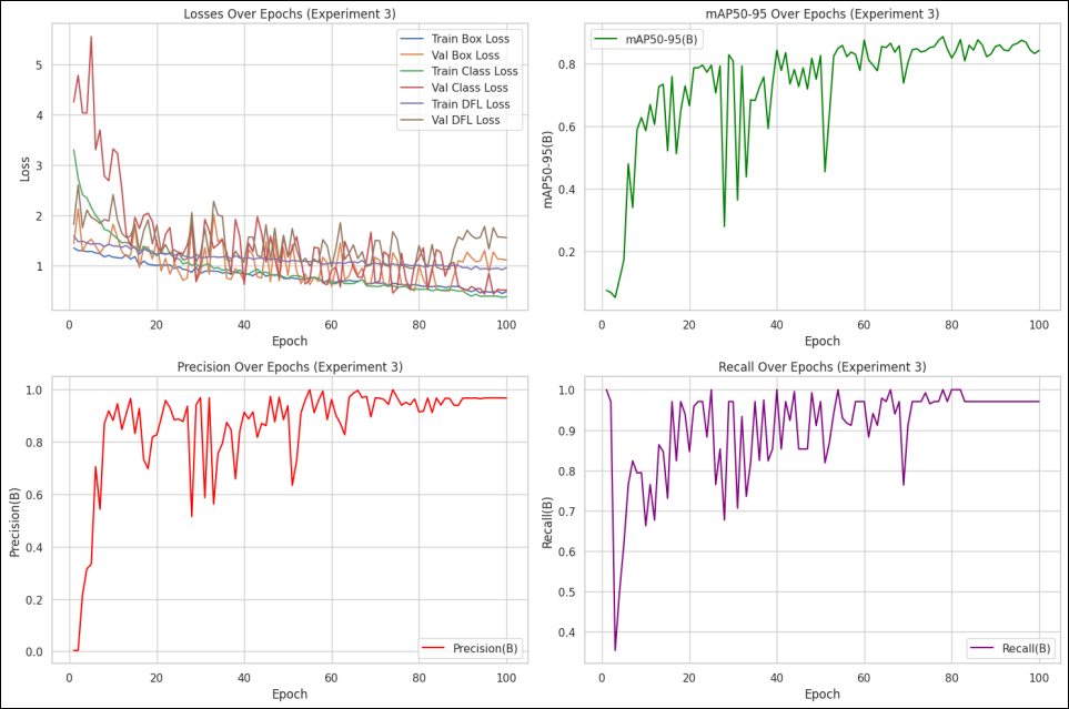
Visão geral — losses, mAP@50-95, Precision e Recall ao longo de 100 épocas (exp3). Mesmo padrão de leve queda entre a melhor época e a final observado no exp1.
