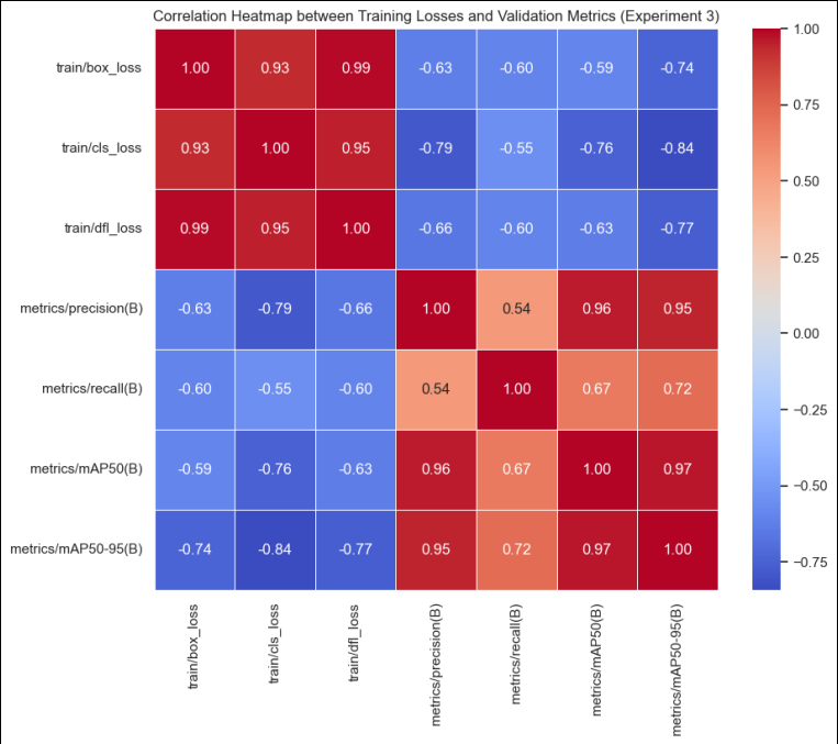
Correlação entre as losses de treino e as métricas de validação (exp3): cls_loss é a mais fortemente (anti)correlacionada com mAP@50-95 (-0,84).
