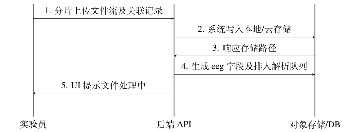
图 11: 上传 EEG 数据文件请求响应时序图
