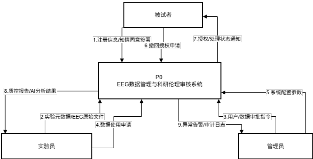
图 14: 顶层数据流图
