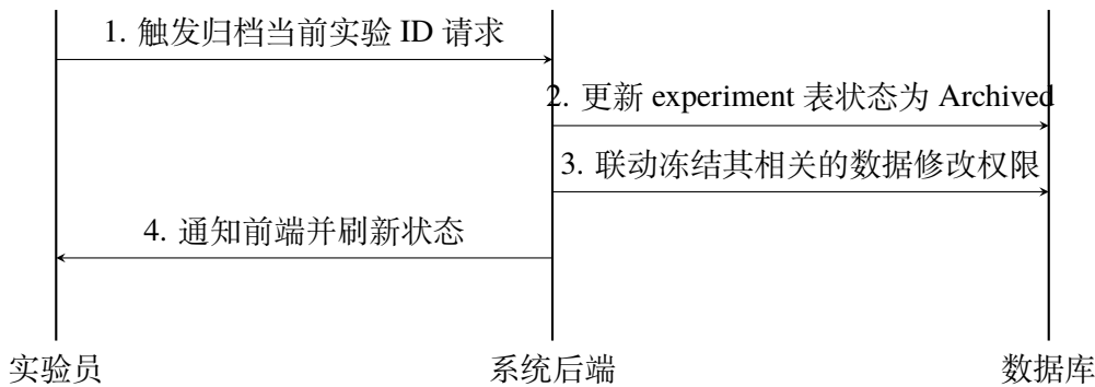
图 8: 归档 EEG 实验请求响应时序图
