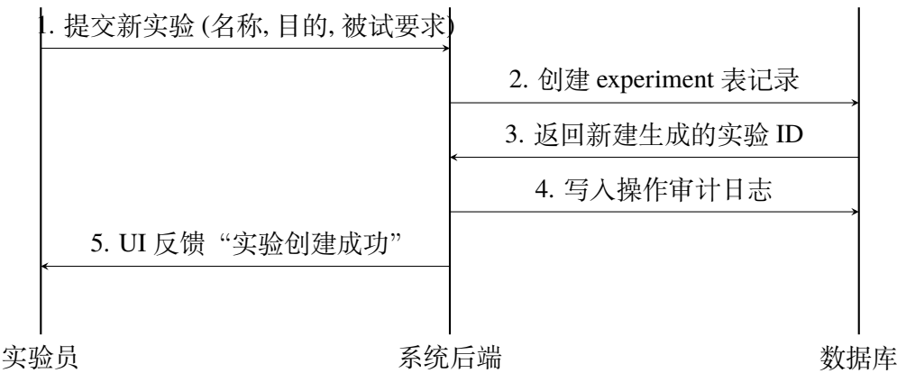
图 7: 创建 EEG 实验请求响应时序图
