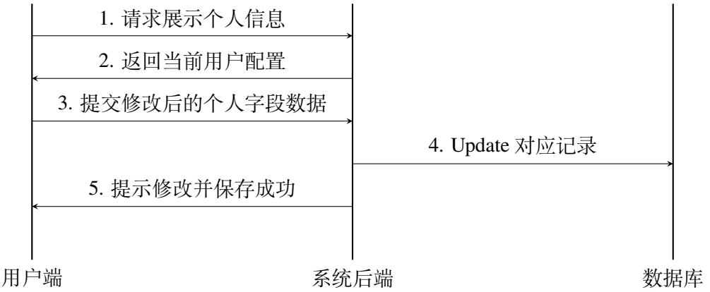
图 6: 个人信息修改请求响应时序图
