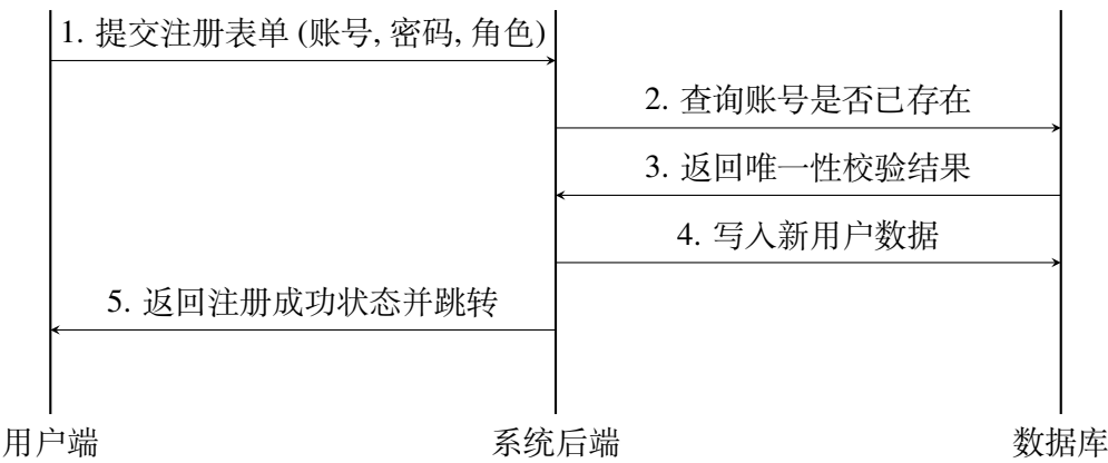
图 4: 用户注册请求响应时序图
