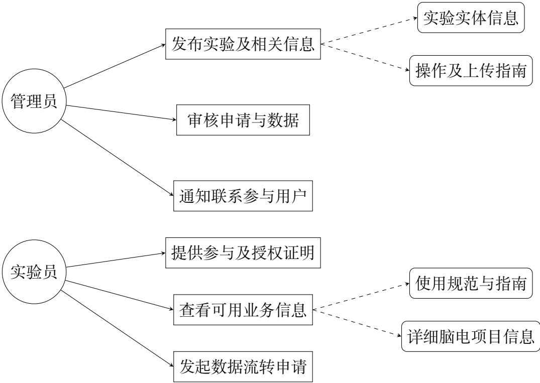
图 2: EEG 实验与申请模块用例图
