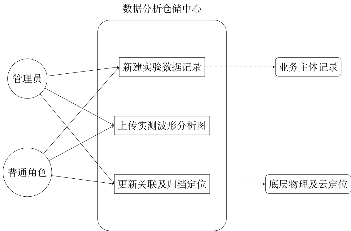
图 3: 数据仓储定位模块用例图
