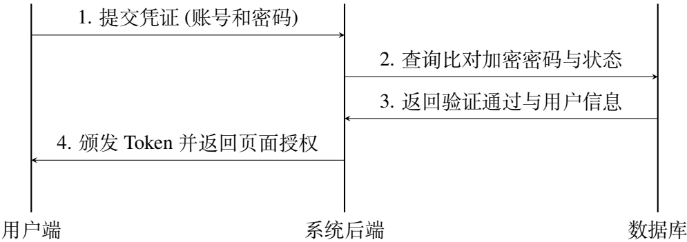
图 5: 用户登录请求响应时序图
