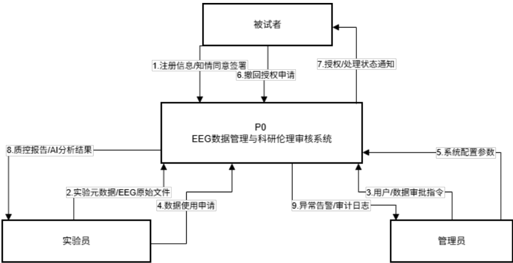
图 12: 顶层数据流图
