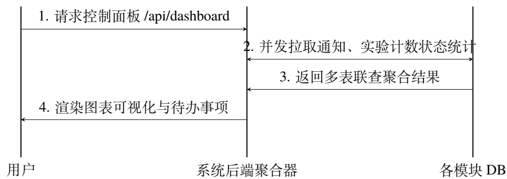
图 11: Dashboard 首页数据请求响应时序图
