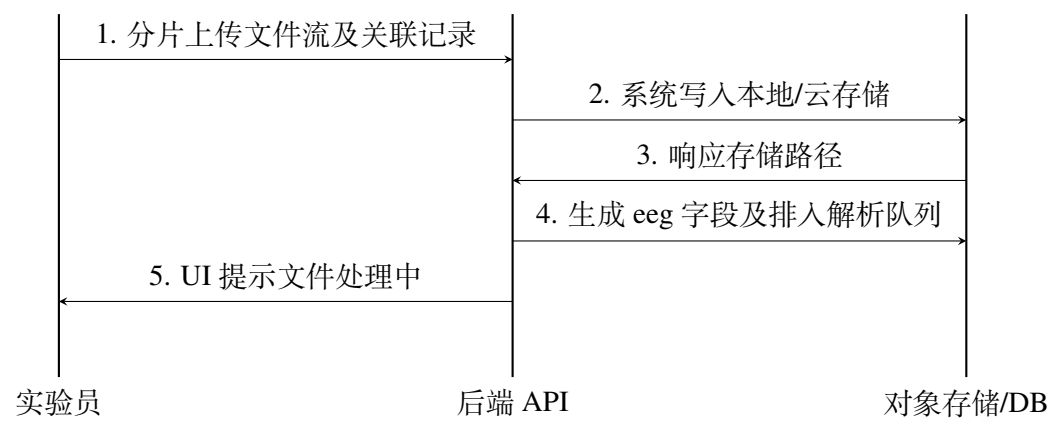
图 9: 上传 EEG 数据文件请求响应时序图
