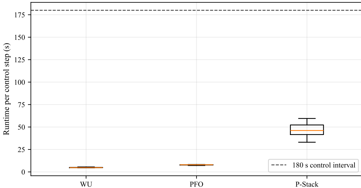
Fig. 6A. Runtime Per Control Step
