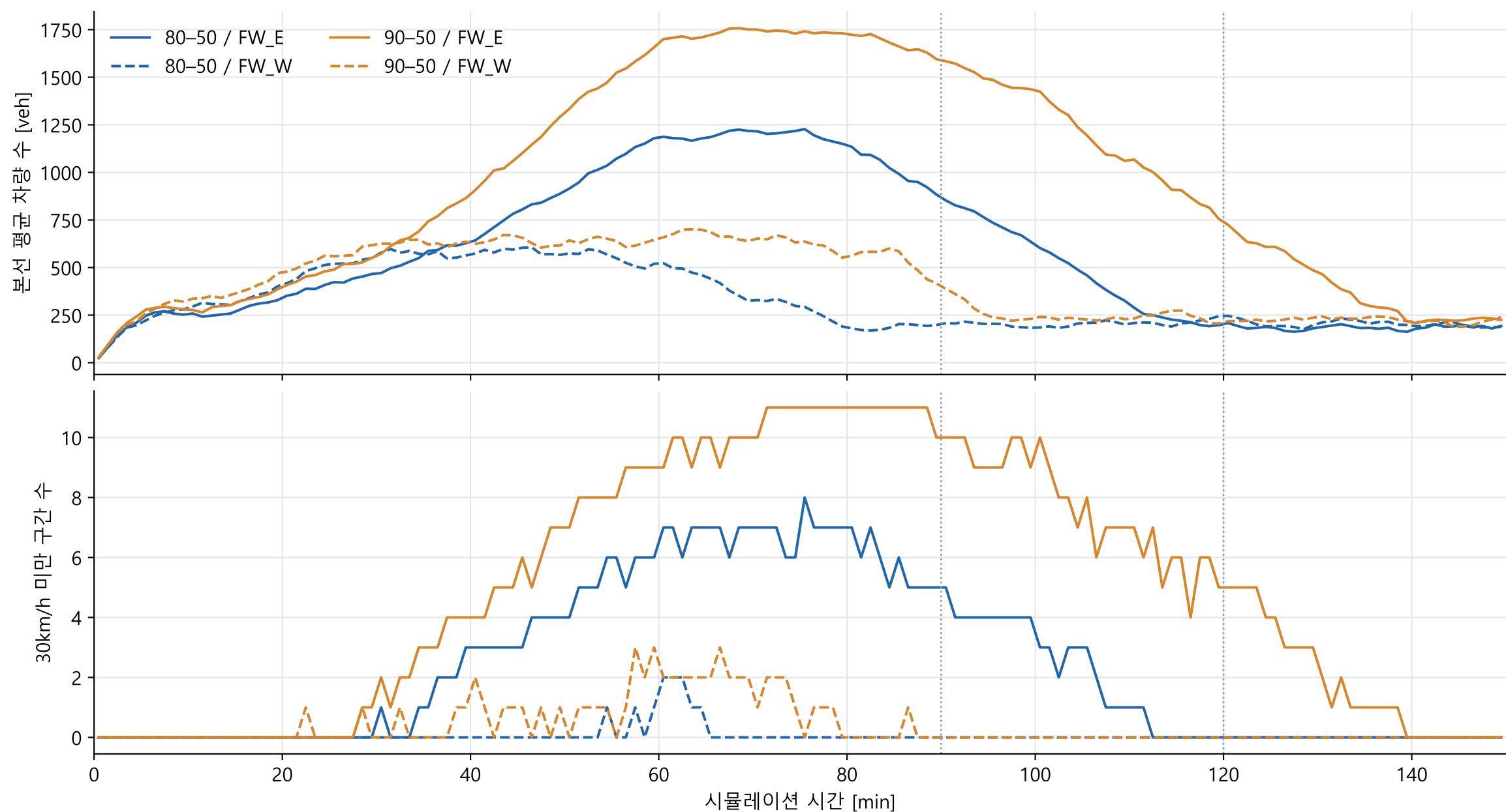
5400초 이후에도 수요를 유지했을 때의 본선 축적·저속 구간
