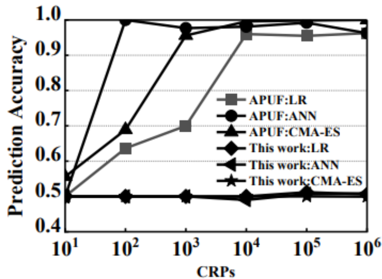
圖二、邏輯層混淆架構之抗攻擊效能分析 [7]
