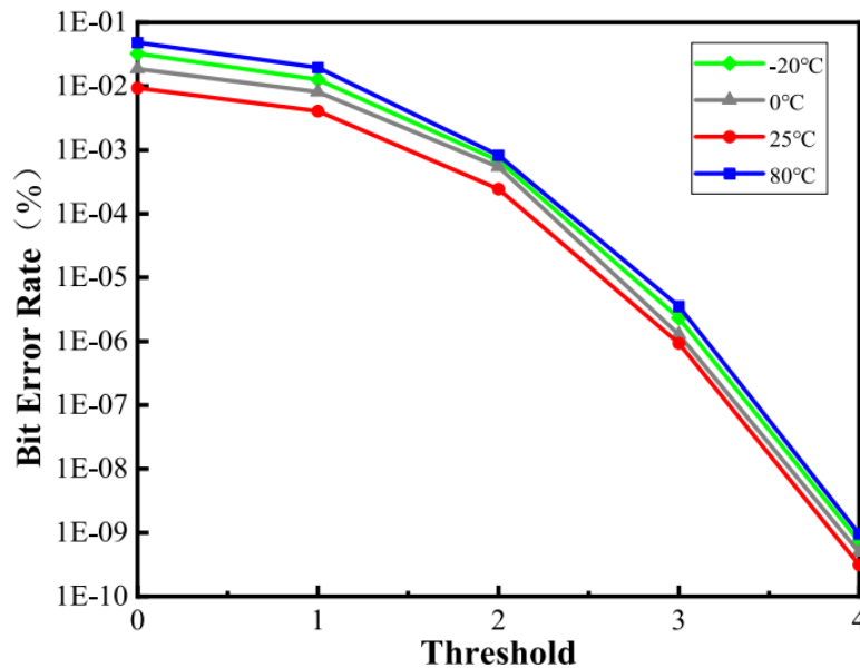
圖一、不同溫度條件下 FPGA RO-PUF 的位元錯誤率 (BER) 變化趨勢 [3]。
