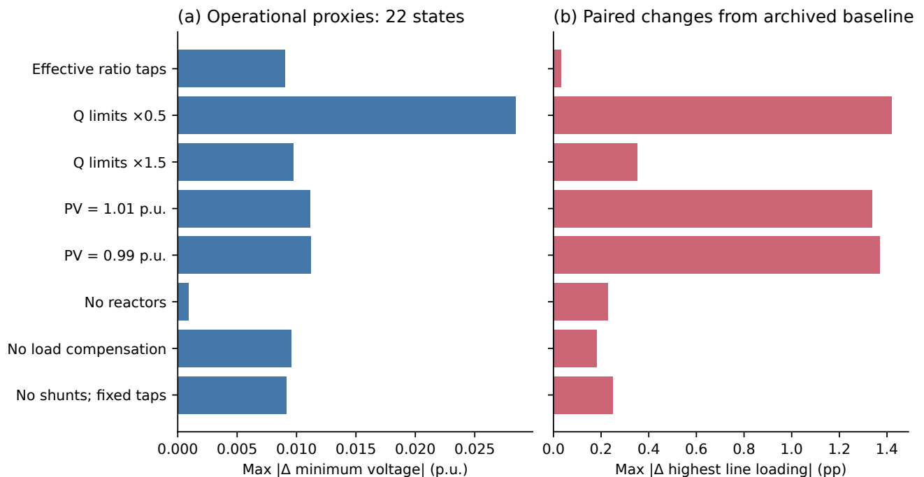
Figure 6——运行代理消融的成对响应。两面板分别表示相对同一时点归档基线的最低电压和最大线路负载率的最大绝对变化，采用 22 个时点与固定的扰动幅度。Table 13 给出全部配置及变压器结果；分接器启用是显式独立变体。
