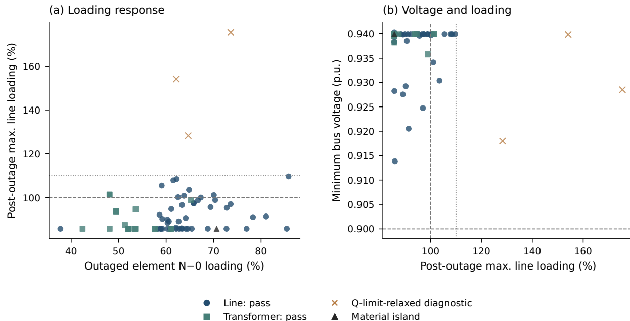
Figure 13——审计后的定向交流 N-1 响应。(a) 被停运元件 N-0 负载率与事故后最高线路负载率；(b) 事故后最高负载率与最低电压。圆点与方点分别为通过筛查的线路和变压器停运案例；叉号为取消无功限值后的诊断解，不计作通过；三角形为实质孤岛。虚线表示 100% 连续定额和 0.90 p.u. 电压下限，点线为仅适用于相应 60 kV 线路的 110% 应急参考，不能据全网最大值单独重判案例类别。70 个案例中 67 个主解收敛，3 个仅有诊断解；数量汇总见 Table 18。归档结果包含 2 个负荷调整、1 个风电削减及 1 个基于公开容量的转供代理案例，不是完全无操作的 N-1 实验。
