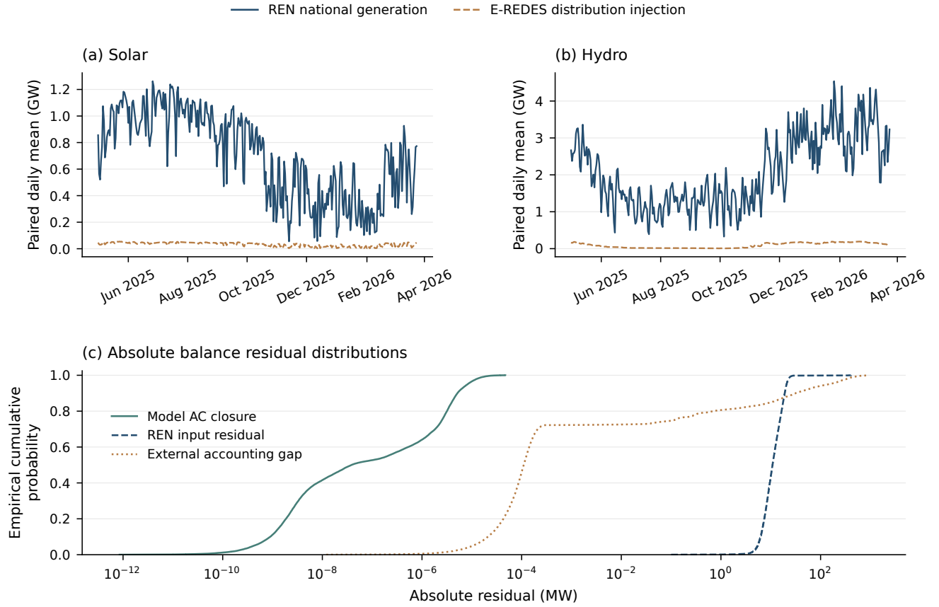
Figure 10——发电统计范围与平衡定义。(a – b) 光伏和水电在成对可用时间戳上的日平均值，区分 REN 全国生产与 E-REDES 配网注入；风电已在 Figure 8 展示，不重复。(c) 三种绝对平衡残差的经验累积分布，分别为模型 AC 闭合 ( n = 31,492 )、REN 输入残差 ( n = 31,492 ) 及外部会计差 ( n = 31,388 )。横轴为对数 MW；REN 残差中 1 个精确零值保留在分母内，不赋予人为正值。三种定义不同，不能作为同一误差排行榜；曲线仅由归档区间值计算，没有拟合或平滑。
