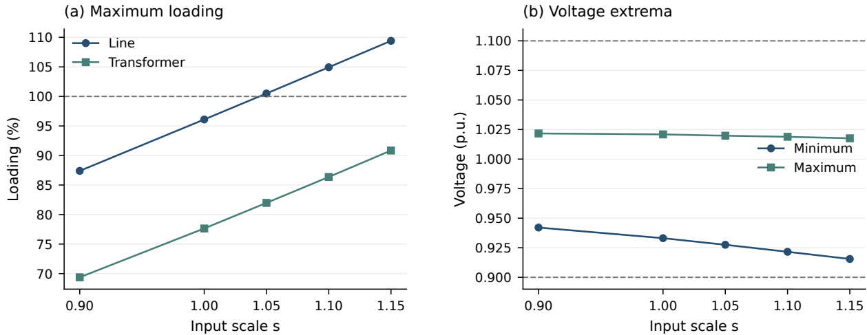
Figure 12——确定性网络压力响应。(a) 最高线路与变压器负载率，虚线为 100% 连续定额；(b) 最低与最高母线电压，虚线为 0.90 – 1.10 p.u. 筛查范围。2026-01-20 19:45 UTC 基准下负荷、发电与交换共同缩放，每个标记对应一次实际 AC 求解，连接线仅引导阅读，不代表额外求解、预测或置信区间。越限线路数量见 Table 17。
