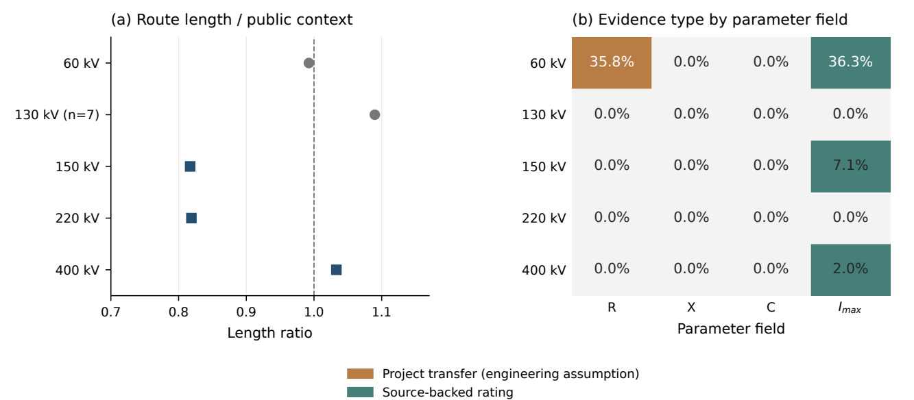
Figure 4——结构覆盖与逐参数来源支撑。(a) 各电压等级的模型 route-km / 公开背景长度比值，虚线为 1；灰色圆点对应非独立 OSM 背景，蓝色方点对应 REN 背景。route-km 与回路长度口径不同，比值不是准确率。(b) 按字段区分项目电阻转用（橙色，工程假设）与有来源定额（绿色），单元格给出对应比例；灰色表示全为工程代理。R 的 35.8% 不是直接参数观测，不能与电流定额的证据等级合并；X、C 均为代理。130 kV 仅 7 条线路，长度比仅供参考。线路级部分支撑计数仍见 Table 10。
