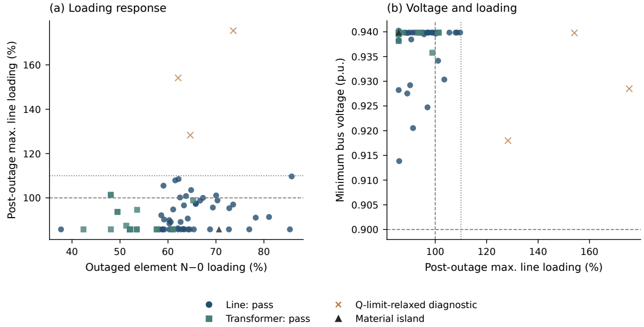
Figure S2——定向交流 N-1 响应。圆点和方点为通过筛查的线路与变压器案例，叉号为仅有诊断解的案例，三角形为实质孤岛；虚线表示连续定额和电压筛查边界。
