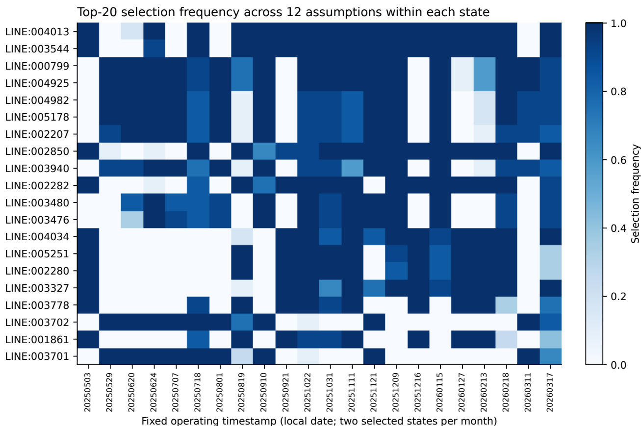
Figure S1——热点线路在不同假设下的入选频率。每格表示一个时点的 12 个配置中进入 Top-20 的比例；完整成员及频率保存在发布 CSV。
