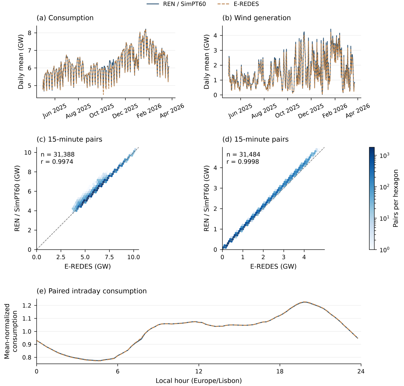
Figure 7——聚合输入的外部时间验证。 (a – b) 全国消费与风电的成对日平均；(c – d) 对应 31,388 与 31,484 个 15 分钟配对，六边形密度共用对数计数色标，虚线为一比一线， r 为 Pearson 系数；(e) 同一消费配对集合按 Lisbon 当地时刻聚合后、各自除以日内均值的曲线。各比较仅排除所需字段缺失的区间，不删除异常月份、不平滑或插值。消费不含抽水和电池充电，与案例总电气负荷区分；风电为全国生产与配网注入的跨范围印证。该图验证聚合输入，不验证节点分配或支路潮流；重采样置信区间 (confidence interval, CI) 见 Table 12。
