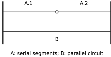
Figure 1——静态网络重建中的连接规则。(a) 同电压端点聚类与设施匹配；(b) 区分几何交叉和显式共享节点；(c) 保留串联分段与并行回路身份；(d) 根据显式资产、同址设施和 RARI 边界证据连接不同电压层。图为抽象电气示意，不表示真实设备坐标；距离阈值及回退规则见 Table 3。
