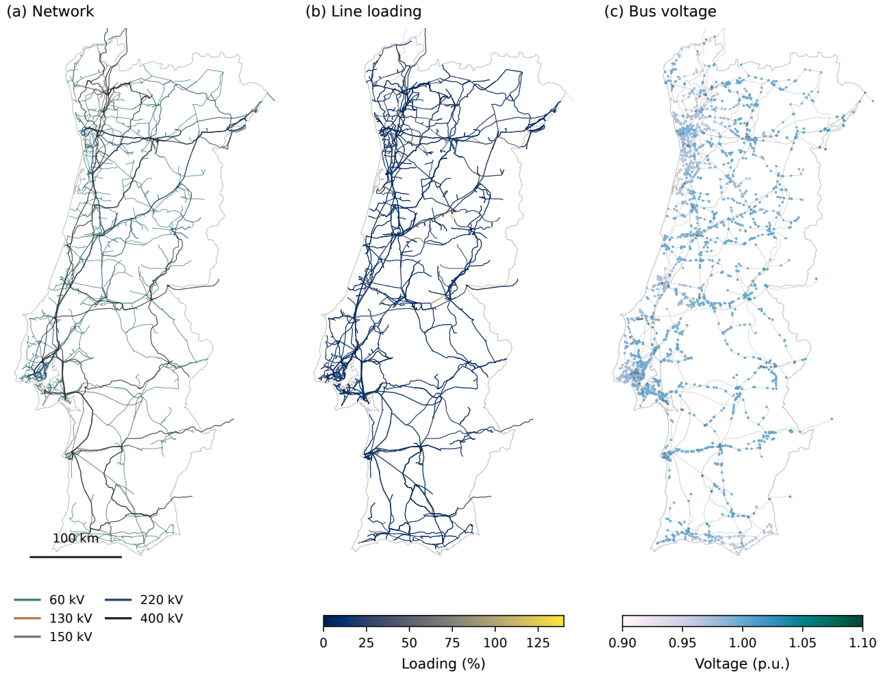
Figure 2——地理网络与年度峰值求解状态。(a) 3,783 个母线、4,943 条线路对应的 60 – 400 kV 地理网络；(b) 线路负载率；(c) 母线电压。三幅地图使用相同 EPSG:3763 投影、空间比例和范围，保留全部原始线路几何及葡西边界端点，比例尺为 100 km。运行状态来自归档的 2026-01-15 12:15 UTC 年度峰值模型（负荷 11,329.2 MW），通过稳定设备 ID 连接；缺失求解状态保留灰色、不填补。色标保留超过 100% 的负载率。结果为模型潮流，不是遥测。
