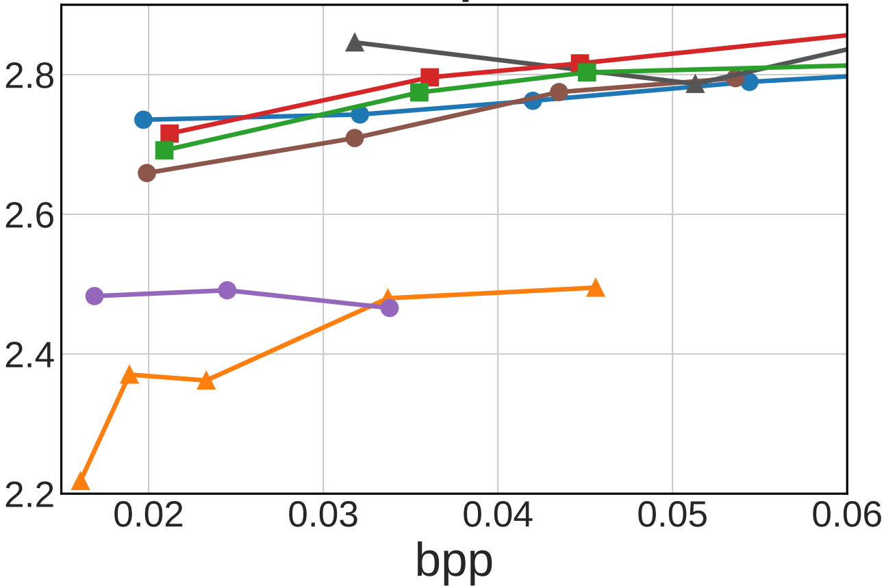
Ewarp ↓
