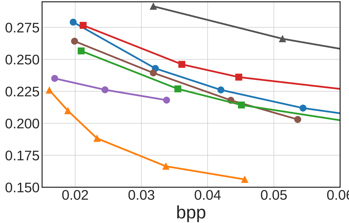
LPIPS ↓
