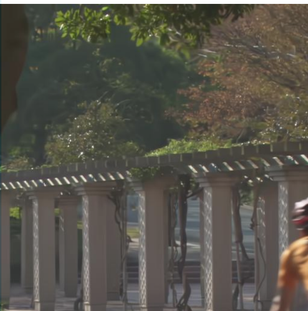
DCVC-FM (0.0288)
