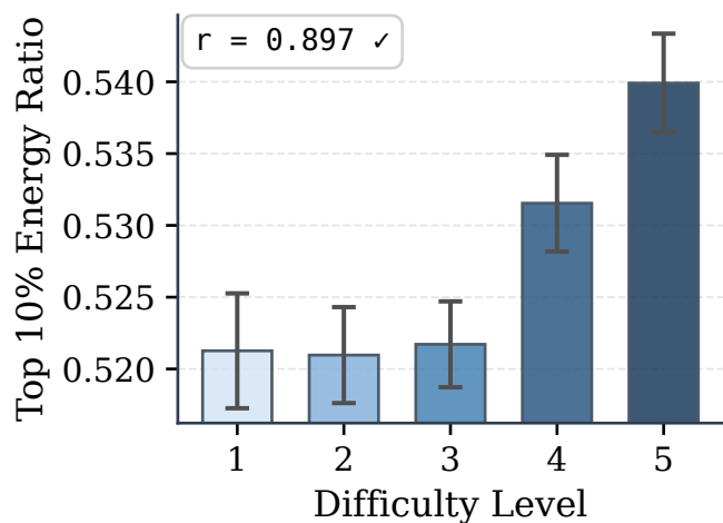
(d) Top 10% Energy Ratio - Llama 3.2 3B
