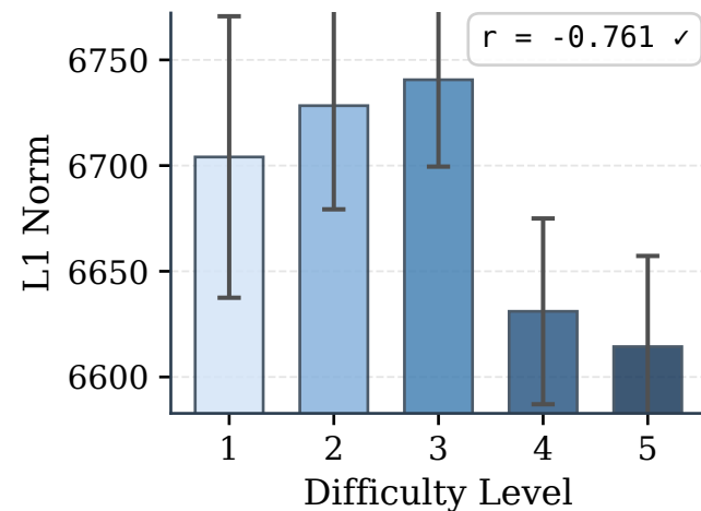
(e) L1 Norm - Llama 3.1 8B
