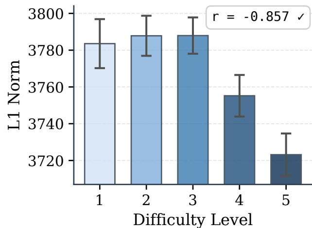
(c) L1 Norm - Llama 3.2 3B
