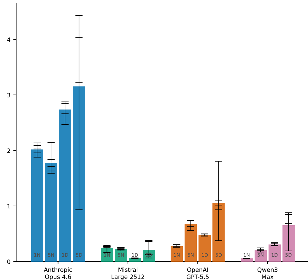
API Cost per run, USD
