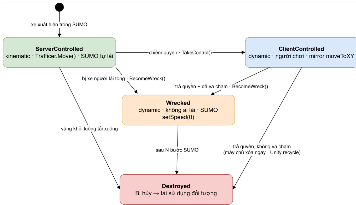
Hình 4.4: Máy trạng thái điều khiển phương tiện
