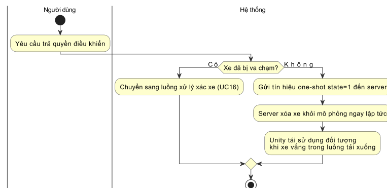
Hình 0.8: Biểu đồ hoạt động use case Trả quyền điều khiển
