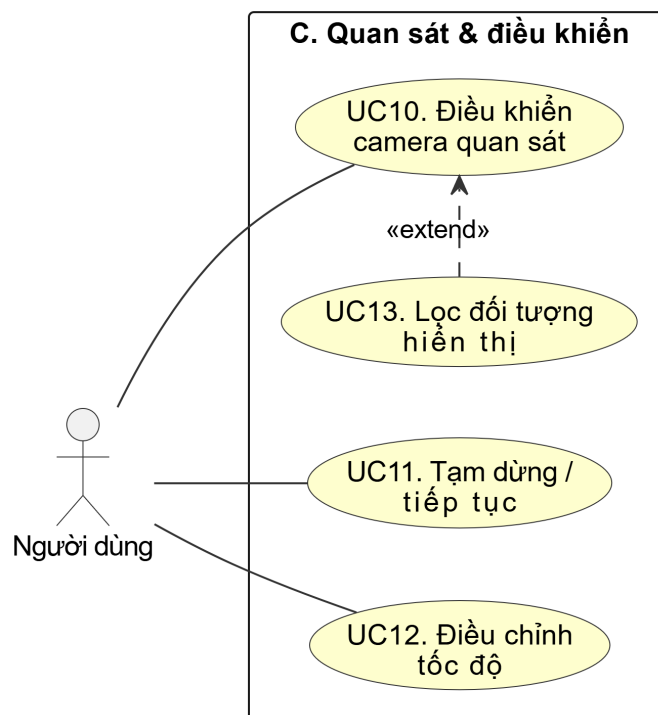
Hình 0.5: Use case nhóm Quan sát và điều khiển
