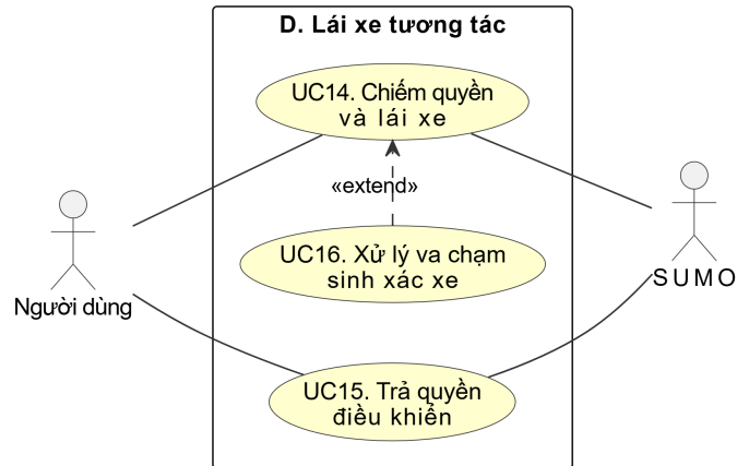
Hình 0.6: Use case nhóm Lái xe tương tác
