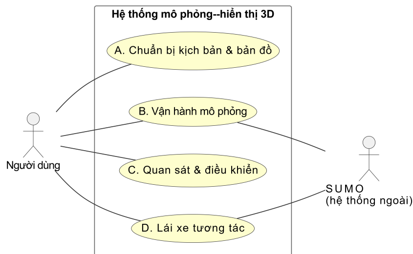
Hình 0.2: Biểu đồ use case tổng quát
