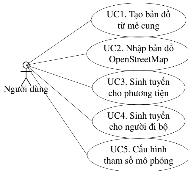
Hình 2.2: Use case nhóm Chuẩn bị kịch bản và bản đồ (bản nháp)
