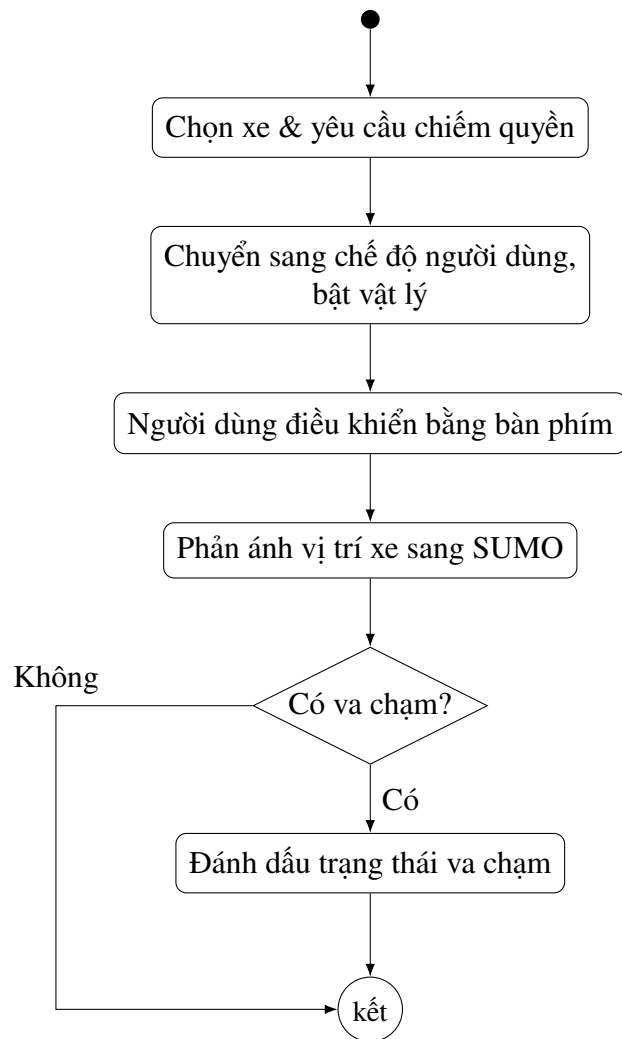
Hình 2.7: Biểu đồ hoạt động use case Chiếm quyền và lái xe (bản nháp)
