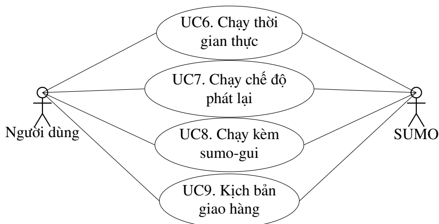
Hình 2.3: Use case nhóm Vận hành mô phỏng (bản nháp)
