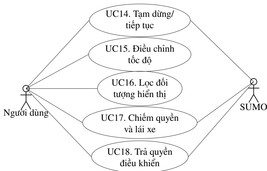
Hình 2.5: Use case nhóm Lái xe tương tác (bản nháp)
