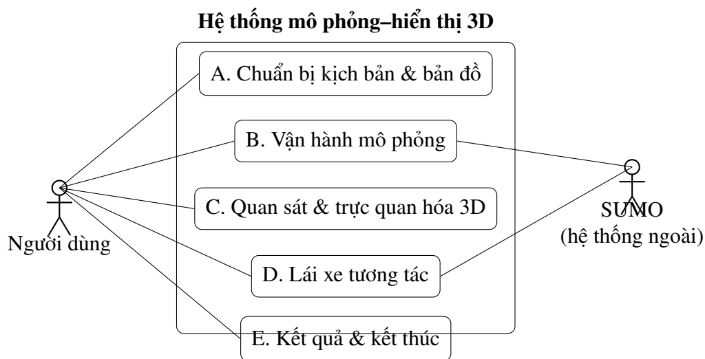
Hình 2.1: Biểu đồ use case tổng quát (bản nháp)
