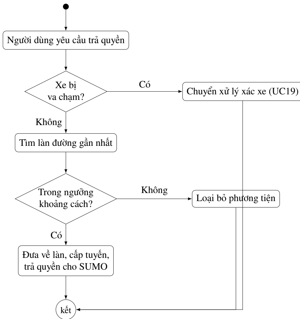
Hình 2.8: Biểu đồ hoạt động use case Trả quyền điều khiển (bản nháp)
