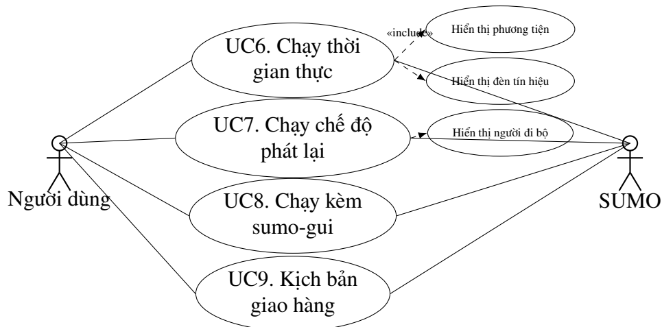
Hình 2.3: Use case nhóm Vận hành mô phỏng (bản nháp)
