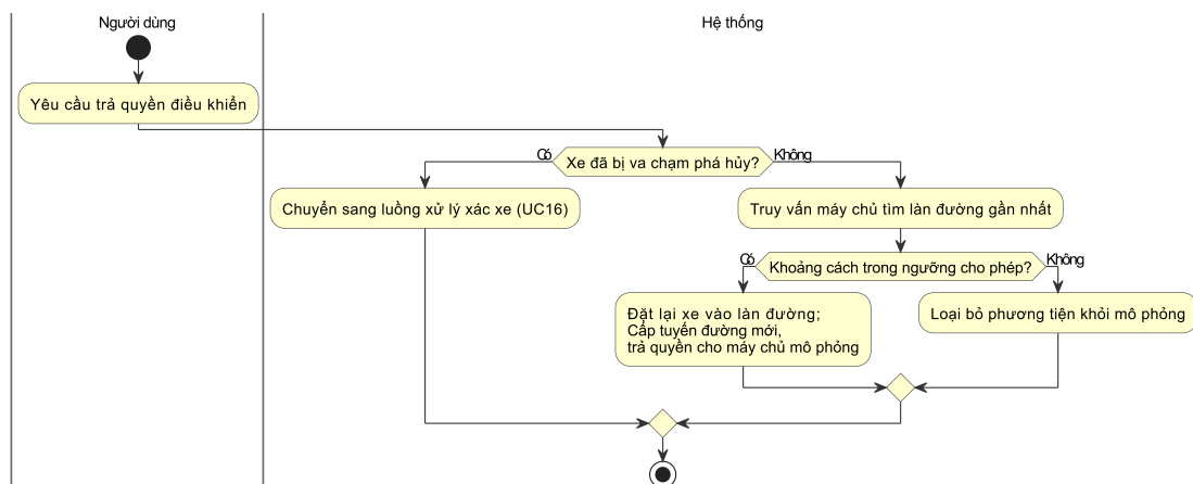
Hình 0.9: Biểu đồ hoạt động use case Trả quyền điều khiển
