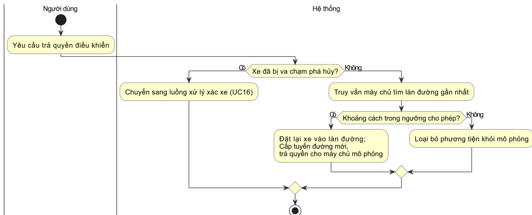
Hình 2.9: Biểu đồ hoạt động use case Trả quyền điều khiển
