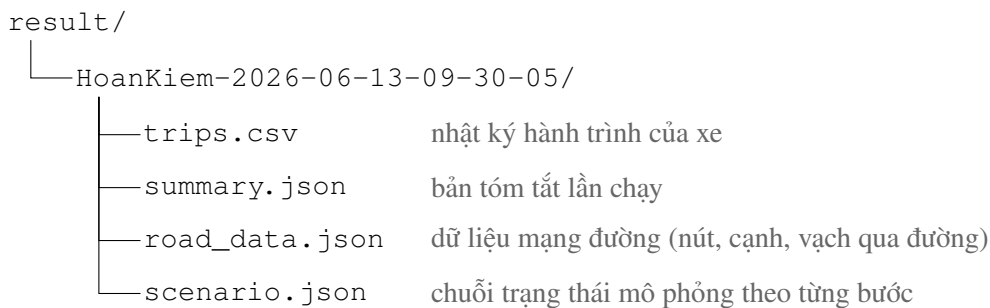
Hình 4.6: Cấu trúc một thư mục phiên tiêu biểu (bản nháp), đặt tên theo bản đồ và thời điểm chạy. Tệp trips.csv đổi thành trips-ped.csv khi kịch bản có người đi bộ.
