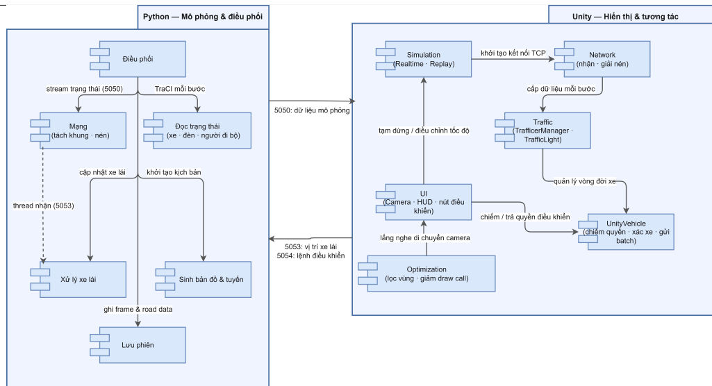
Hình 4.2: Sơ đồ gói các nhóm mô-đun hai phía và quan hệ phụ thuộc
