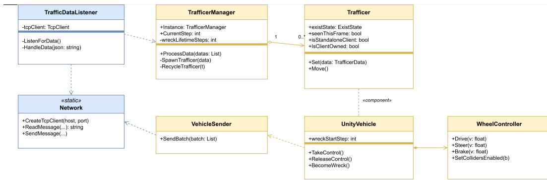
Hình 4.5: Sơ đồ lớp các lớp chủ đạo phía Unity. Lớp SimulationSession thuộc phía Python, không liên kết trực tiếp với nhóm lớp này.
