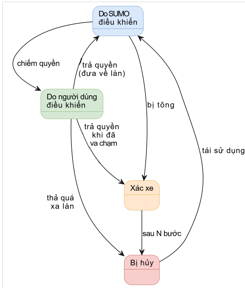
Hình 4.3: Máy trạng thái điều khiển phương tiện
