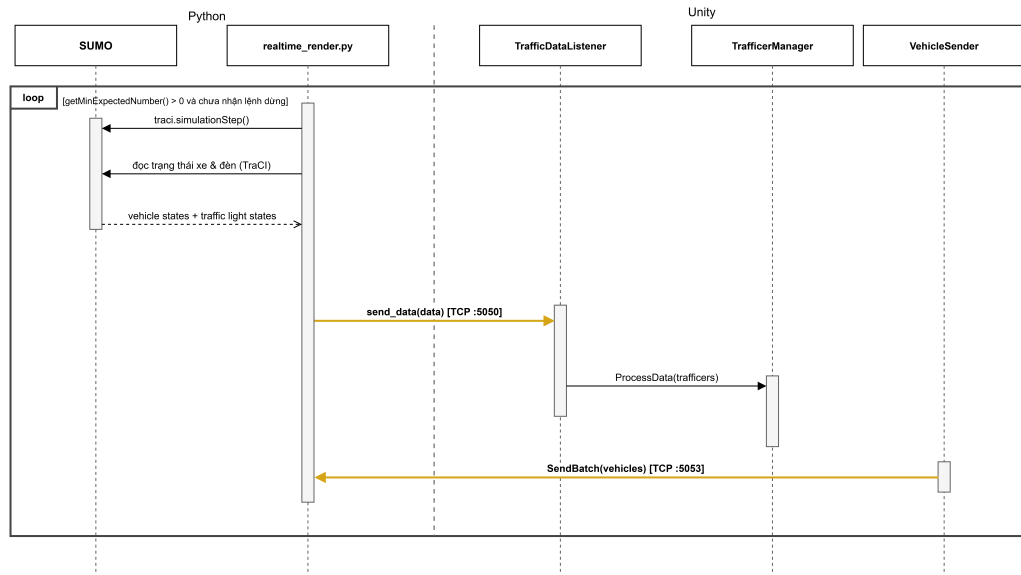
Hình 4.4: Trình tự trao đổi thông điệp giữa mô phỏng và hiển thị trong một bước
