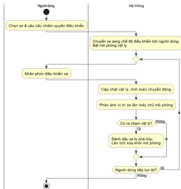
Hình 2.8: Biểu đồ hoạt động use case Chiếm quyền và lái xe
