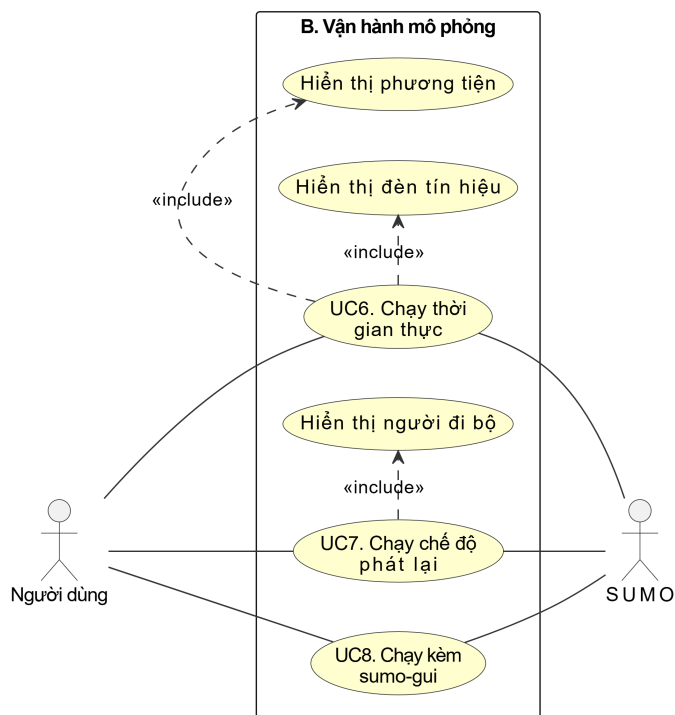
Hình 2.4: Use case nhóm Vận hành mô phỏng
