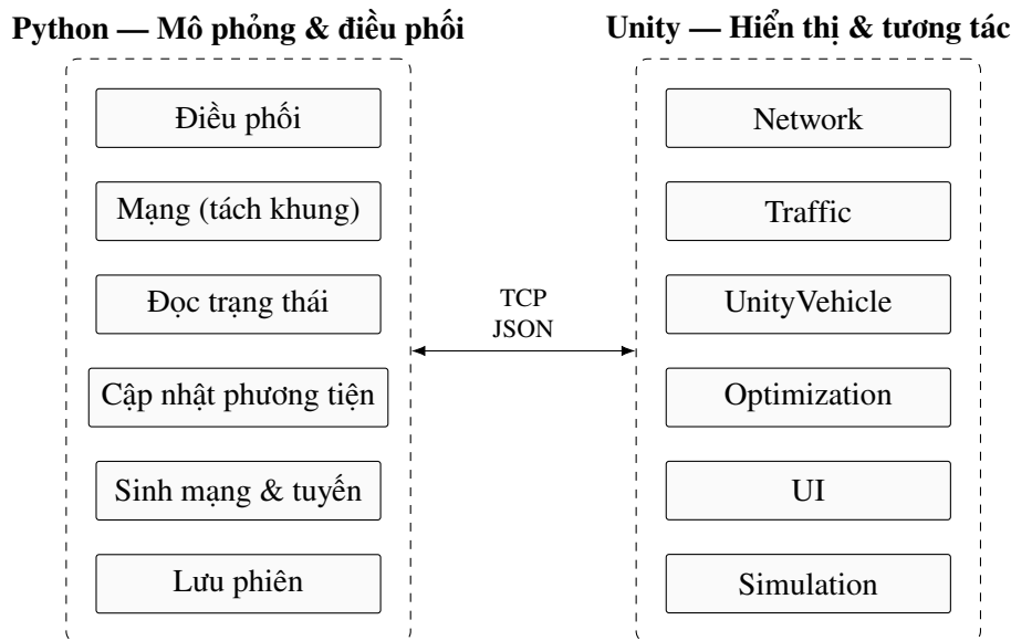
Hình 4.2: Sơ đồ gói các nhóm mô-đun hai phía và quan hệ phụ thuộc (bản nháp)
