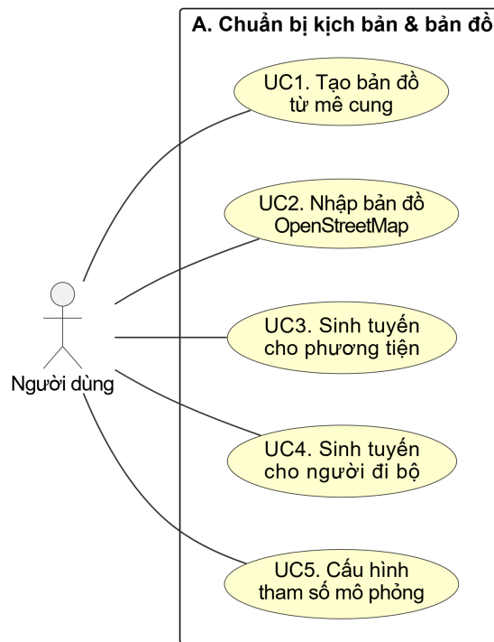
Hình 2.3: Use case nhóm Chuẩn bị kịch bản và bản đồ
