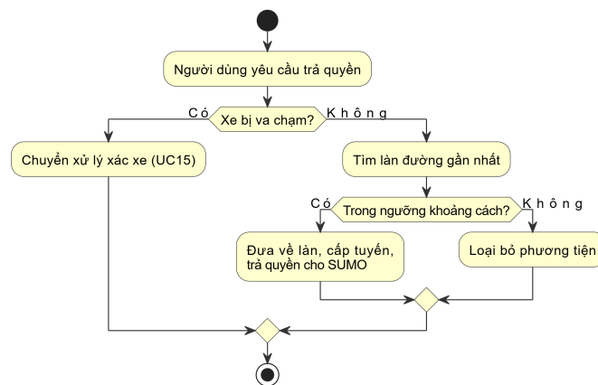
Hình 0.9: Biểu đồ hoạt động use case Trả quyền điều khiển
