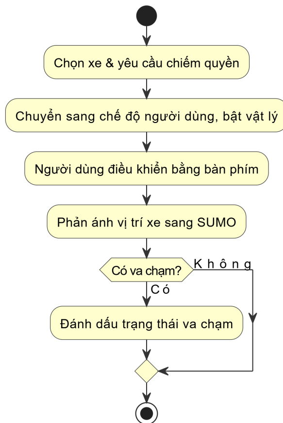
Hình 0.8: Biểu đồ hoạt động use case Chiếm quyền và lái xe
