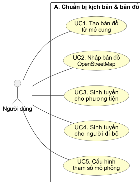
Hình 0.3: Use case nhóm Chuẩn bị kịch bản và bản đồ
