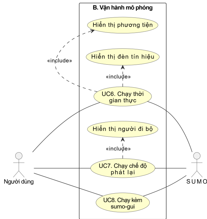
Hình 0.4: Use case nhóm Vận hành mô phỏng
