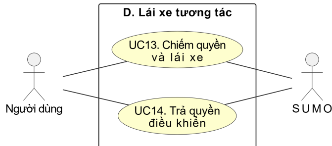
Hình 0.6: Use case nhóm Lái xe tương tác
