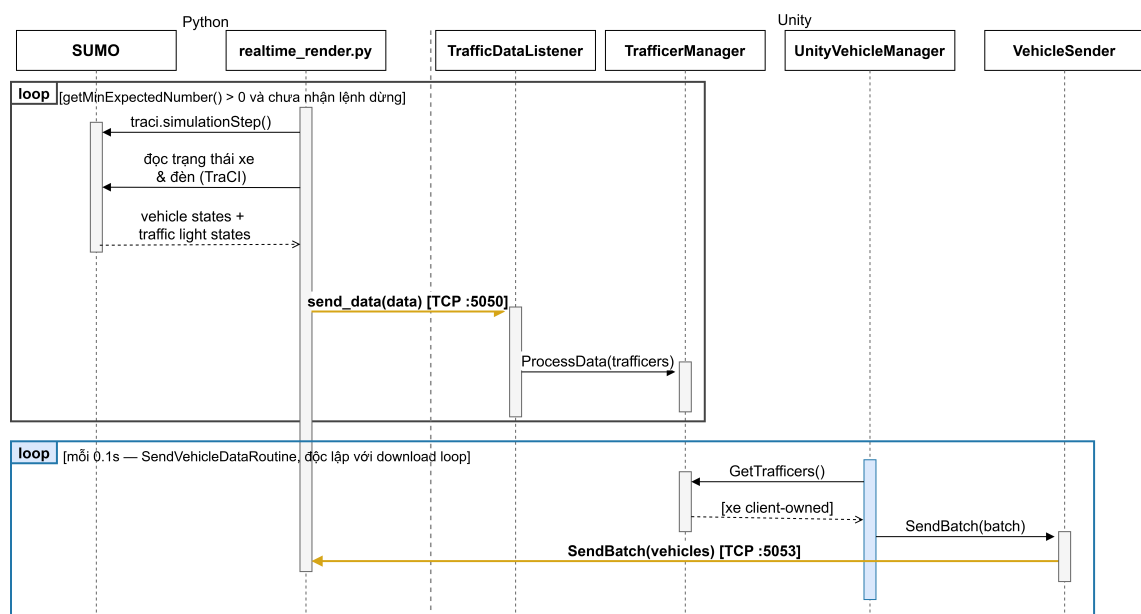
Hình 4.4: Trình tự trao đổi thông điệp giữa mô phỏng và hiển thị trong một bước
