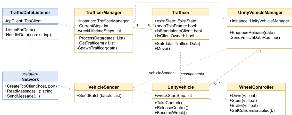
Hình 4.5: Sơ đồ lớp các lớp chủ đạo phía Unity. Lớp SimulationSession thuộc phía Python, không liên kết trực tiếp với nhóm lớp này.
