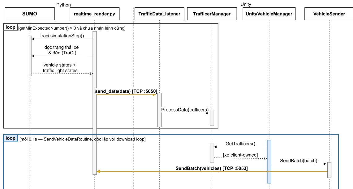
Hình 0.4: Trình tự trao đổi thông điệp giữa mô phỏng và hiển thị trong một bước
