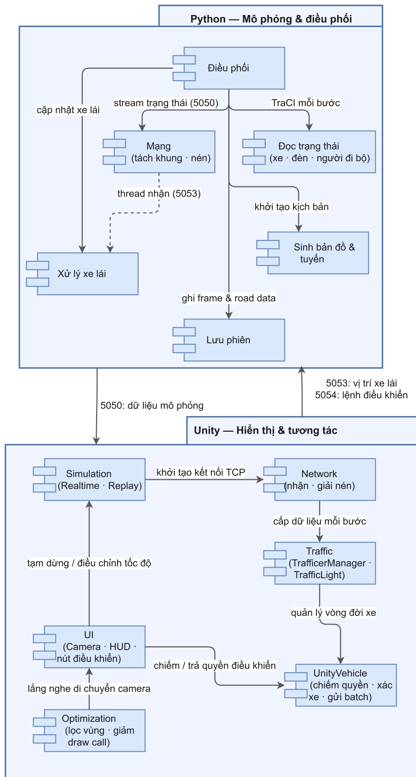
Hình 0.2: Sơ đồ gói các nhóm mô-đun hai phía và quan hệ phụ thuộc
