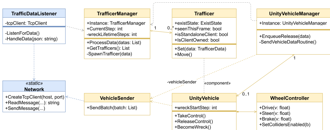
Hình 0.5: Sơ đồ lớp các lớp chủ đạo phía Unity. Lớp SimulationSession thuộc phía Python, không liên kết trực tiếp với nhóm lớp này.
