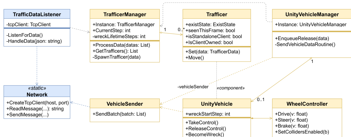
Hình 4.6: Sơ đồ lớp các lớp chủ đạo phía Unity. Lớp SimulationSession thuộc phía Python, không liên kết trực tiếp với nhóm lớp này.
