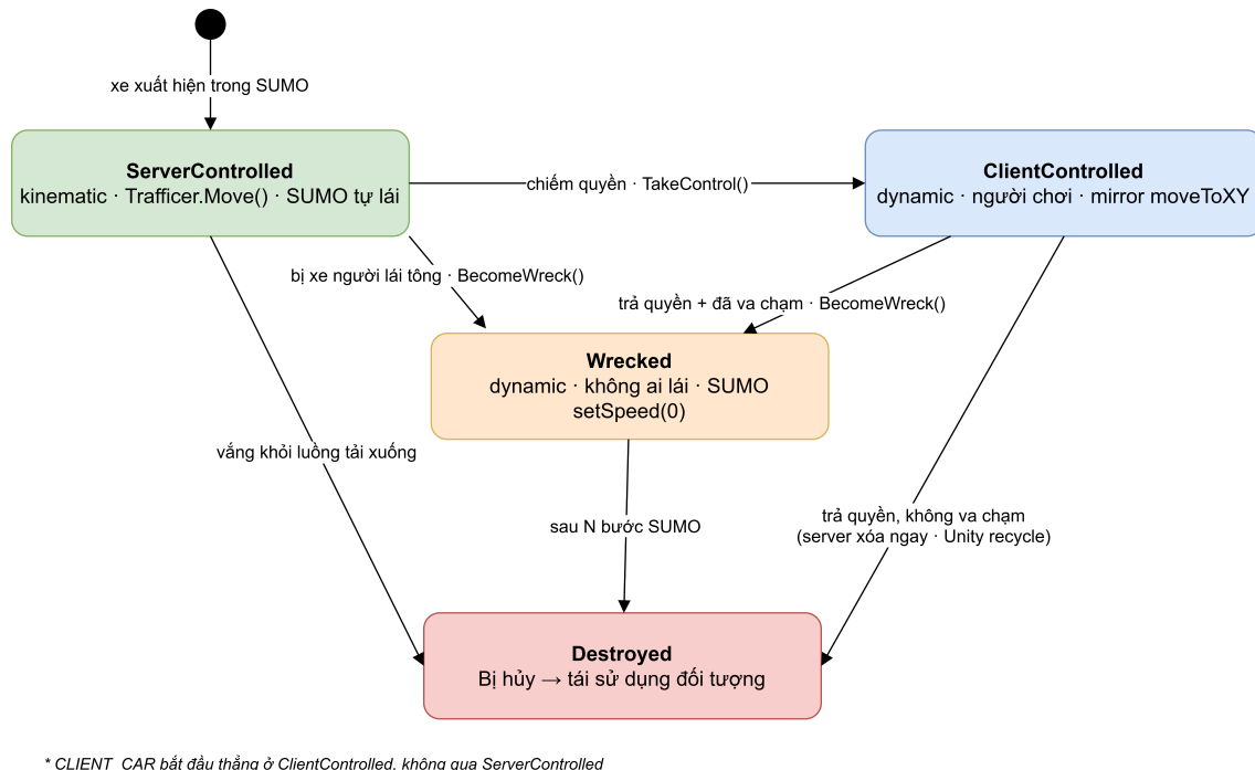
Hình 4.3: Máy trạng thái điều khiển phương tiện
