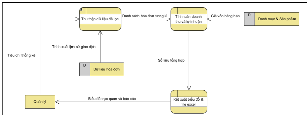
Sơ đồ DFD Mức 1 - Phân hệ Thống kê & Báo cáo doanh thu
