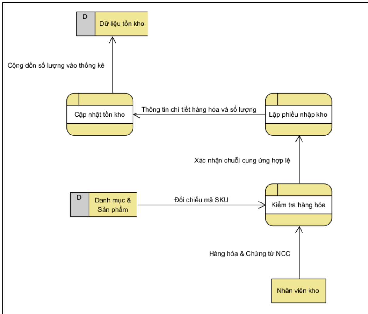
Sơ đồ DFD Mức 1 - Phân hệ 2.0: Quản lý Nhập kho
