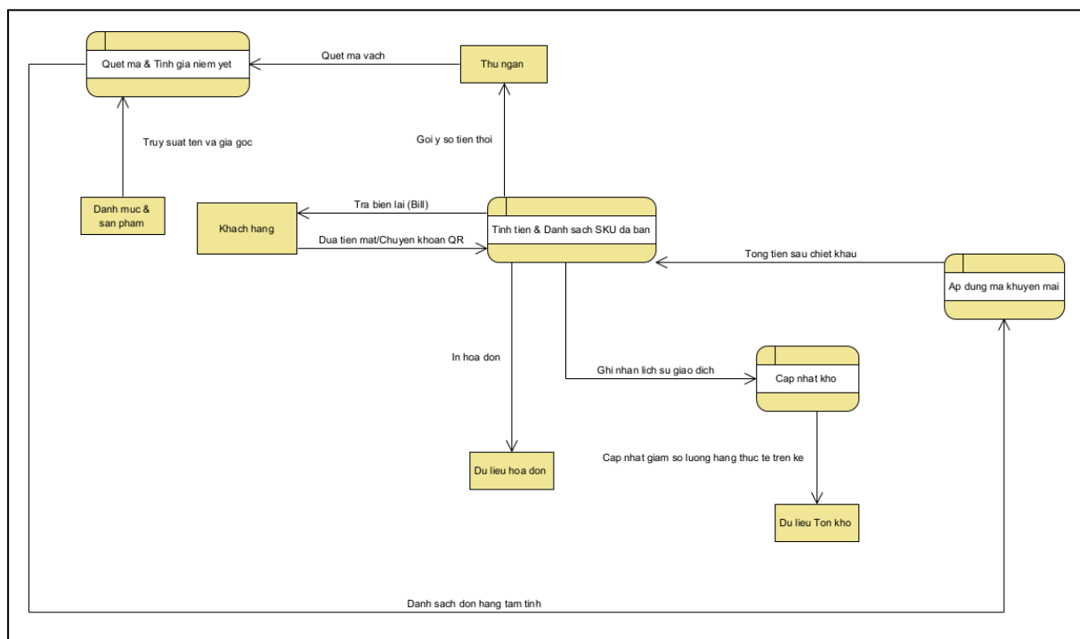
Sơ đồ DFD Mức 1 - Phân hệ 3.0: Quản lý Bán hàng (POS)
