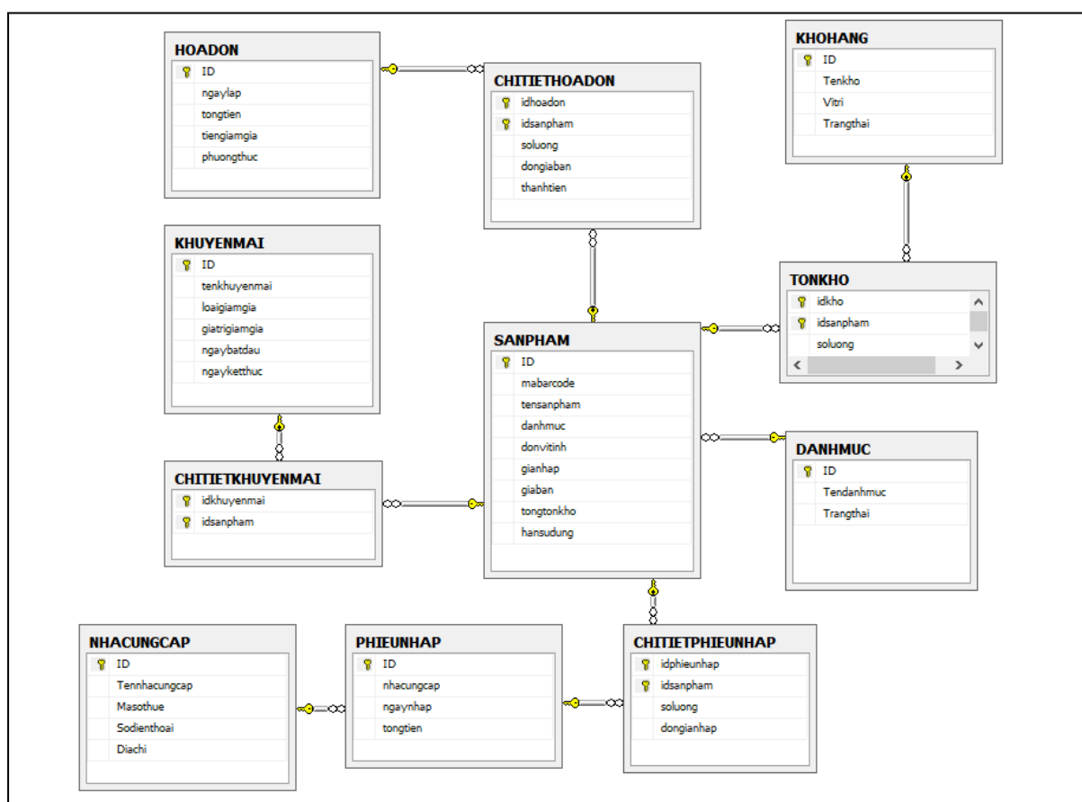
Mô tả tổng quan Lược đồ cơ sở dữ liệu hệ thống
