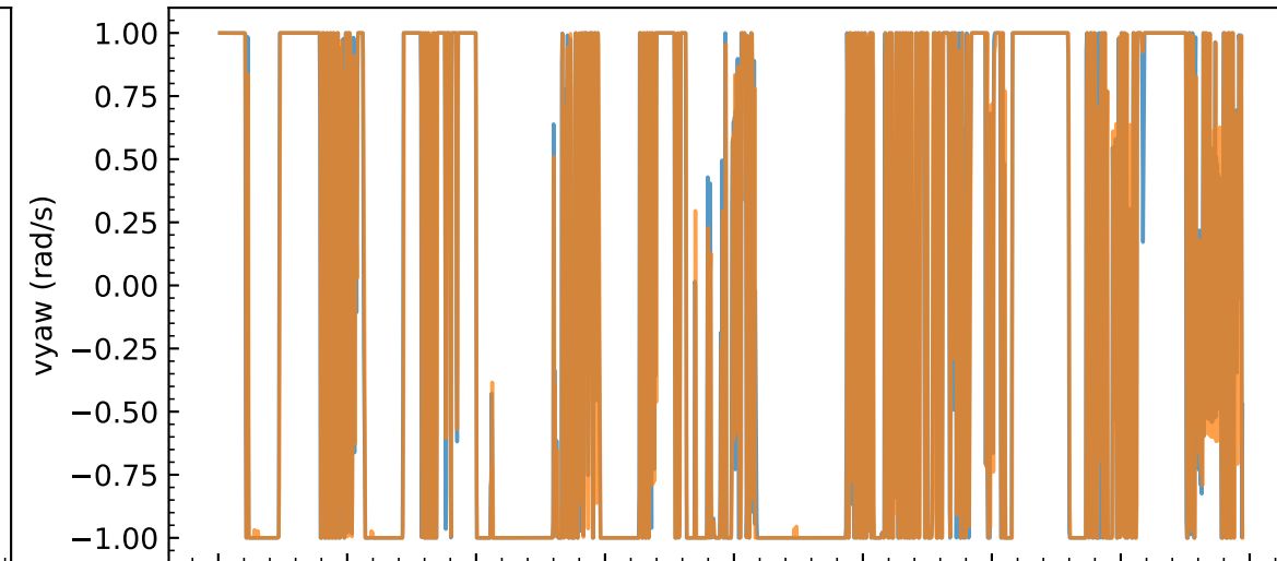
TD3_direct - vyaw: commanded vs actual
