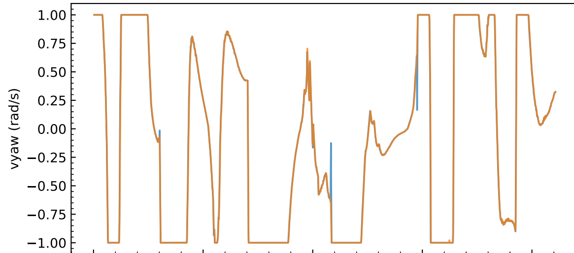
APF - vyaw: commanded vs actual
