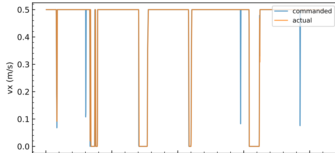
APF - vx: commanded vs actual
