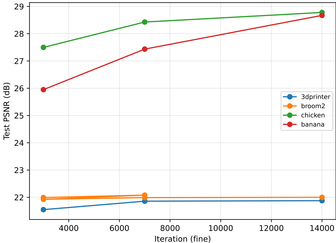
Hội tụ PSNR — hypernerf
