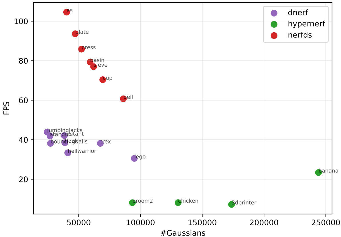
FPS vs #Gaussians (mỗi điểm = 1 scene)
