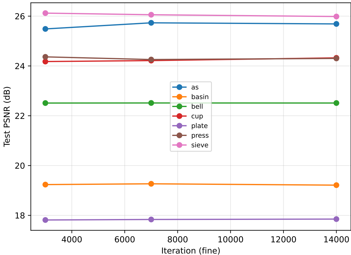
Hội tụ PSNR — nerfds
