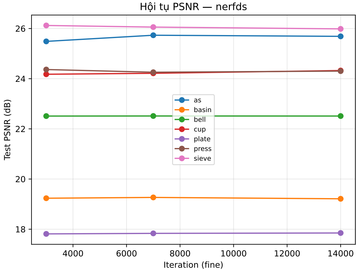
Hình 3.8: Tiến trình PSNR test của 7 cảnh NeRF-DS theo vòng lặp giai đoạn fine (eval tại 3.000/7.000/14.000). Số liệu từ log huấn luyện (tensorboard, tập test lấy mẫu), dùng đọc xu hướng; có thể lệch nhẹ so với số metrics.py ở bảng per-scene.
