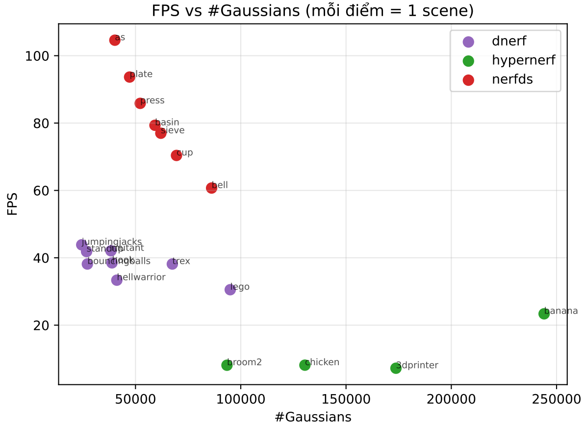
Hình 3.11: Quan hệ tốc độ render (FPS) và số Gaussian mỗi cảnh; mỗi điểm là một cảnh (cùng kiểu phân tích với hình point-FPS của bài báo gốc). FPS giảm khi số Gaussian tăng, lý giải vì sao cảnh quy mô lớn sẽ phá vỡ tính thời gian thực.
