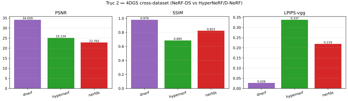
Hình 3.10: So sánh 4D-GS trên ba dataset (PSNR/SSIM/LPIPS). PSNR giảm dần theo trục tổng hợp (D-NeRF) → thật (HyperNeRF) → thật phản chiếu (NeRF-DS); riêng SSIM/LPIPS không đơn điệu do khác độ phân giải và cảnh (xem phần “Độc kết quả”).
