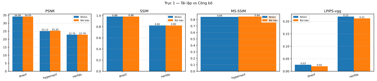
Hình 3.9: Trục 1: đối sánh kết quả nhóm với số công bố trên từng dataset (D-NeRF: PSNR/SSIM/LPIPS; HyperNeRF: PSNR/MS-SSIM; NeRF-DS: PSNR/SSIM/LPIPS-vgg so SpectroMotion [12]). Cột “Nhóm” sát cột “Bài báo” xác nhận tái lập đúng.
