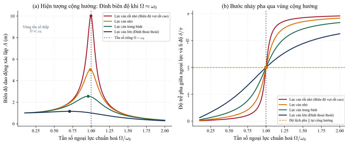
Hình 6: Đường cong cộng hưởng biên độ đạt đỉnh khi tần số ngoại lực trùng khớp với tần số riêng.
