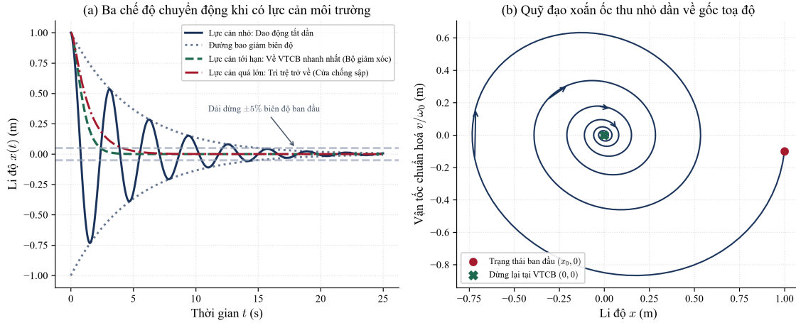
Hình 5: Ba chế độ chuyển động khi có lực cản môi trường và đồ thị trạng thái xoắn ốc.
