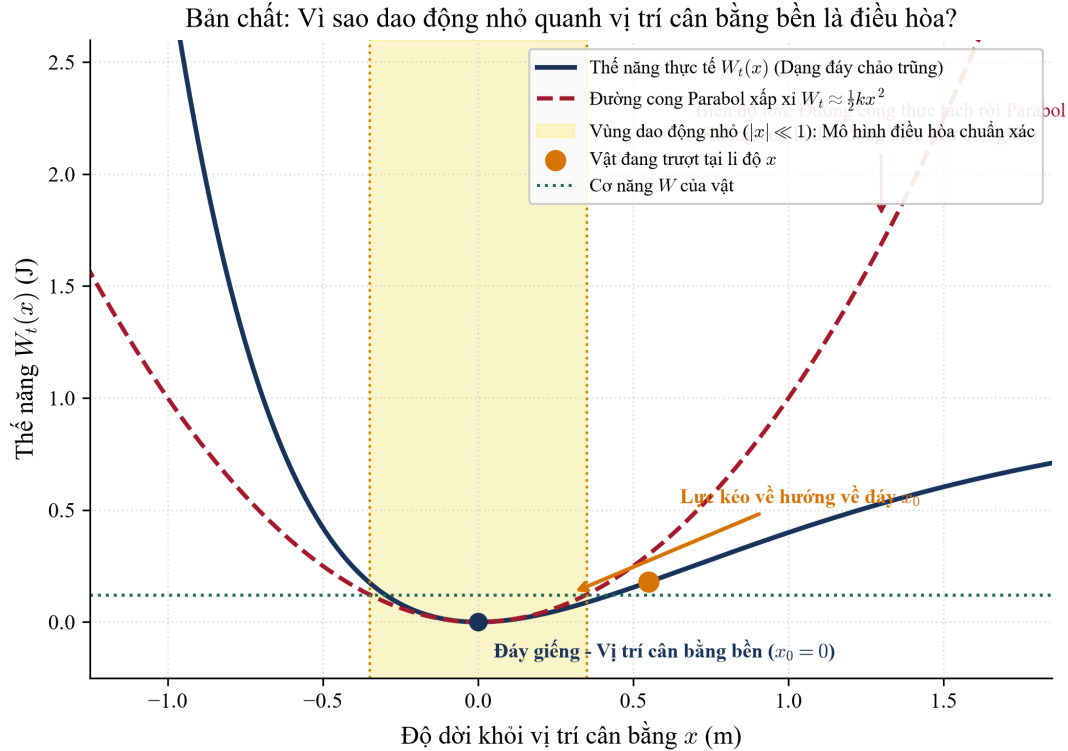
Hình 3: Bản chất hình học của đáy giếng thế năng: Dao động nhỏ quanh vị trí cân bằng bền luôn có thể năng dạng Parabol.
