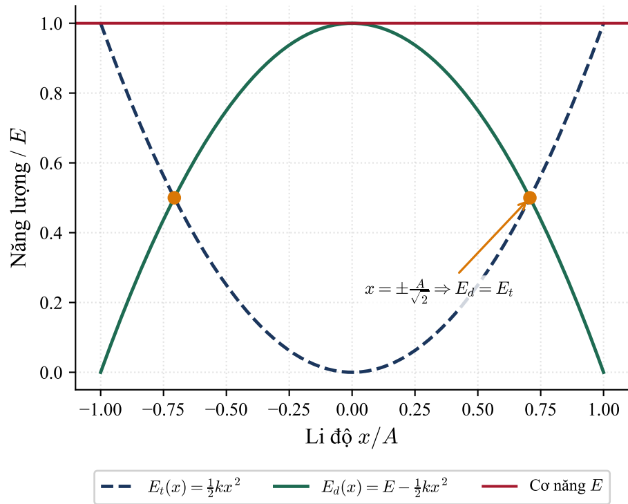
(b) Phân bố năng lượng theo li độ
