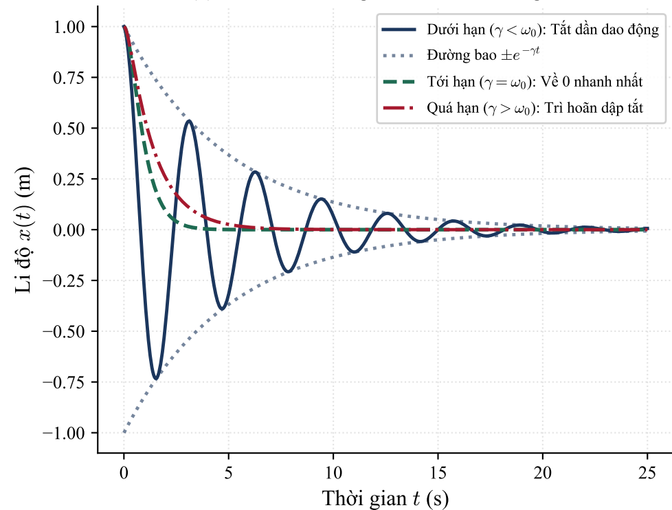
(a) Ba chế độ động học của dao động cản
