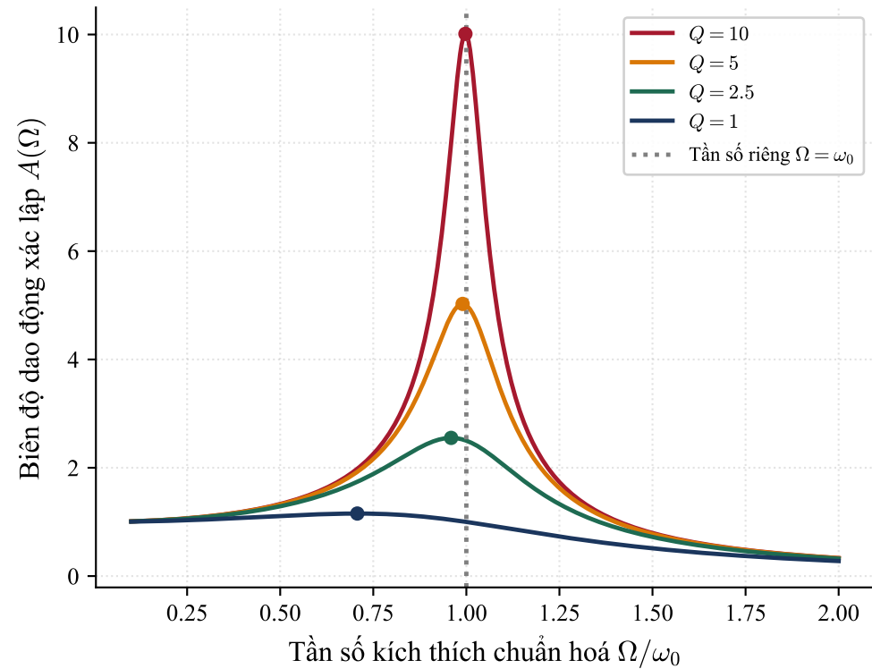
(a) Đường cong cộng hưởng biên độ
