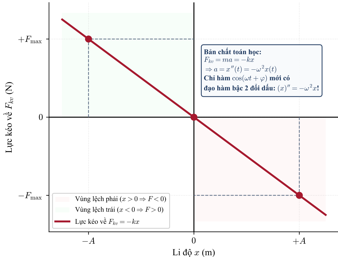
(b) Đồ thị Lực kéo về: Luôn ngược dấu với li độ
