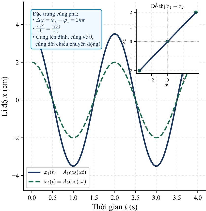
(a) CÙNG PHA: \Delta\varphi = 2k\pi
