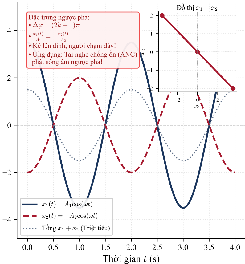
(b) NGƯỢC PHA: \Delta\varphi = (2k + 1)\pi
