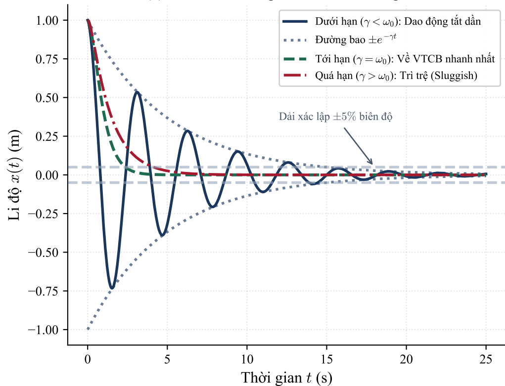
(a) Ba chế độ động học của dao động cản
