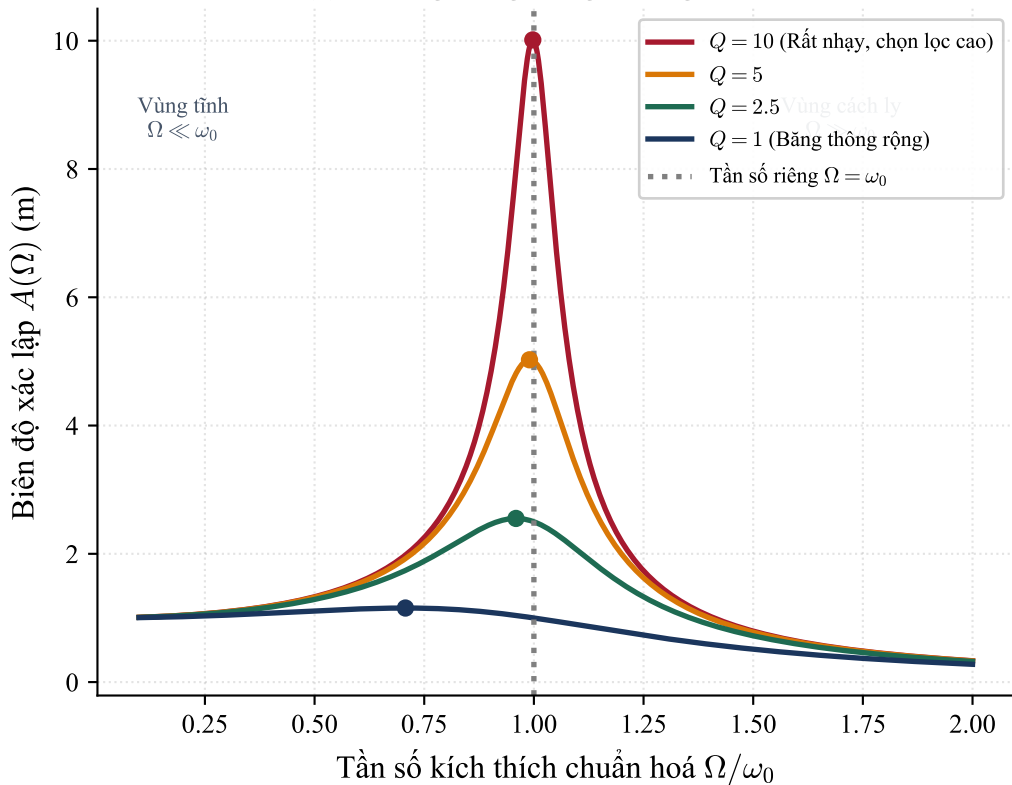
(a) Đường cong cộng hưởng biên độ
