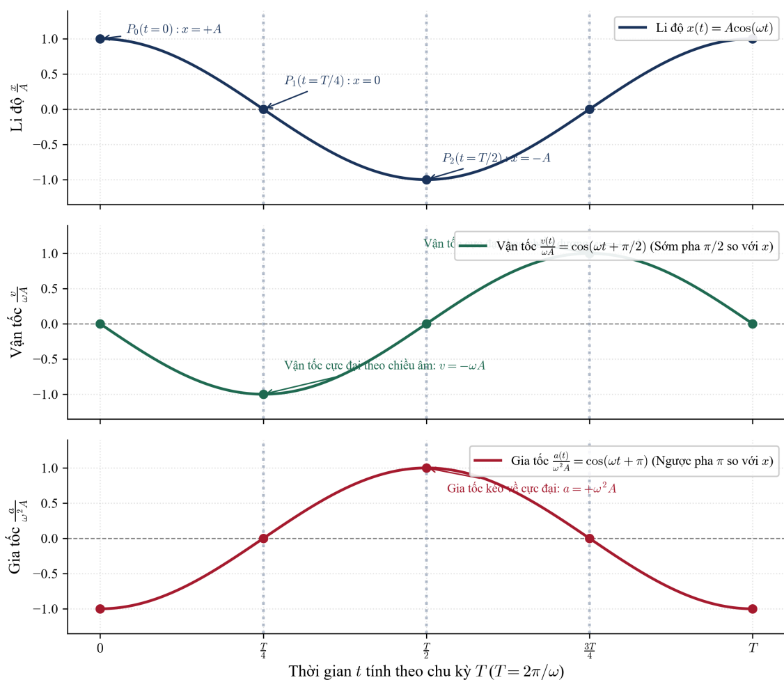
Hình 2: Đồ thị động học chuẩn hóa theo thời gian của dao động điều hòa: Li độ x(t) , Vận tốc v(t) , và Gia tốc a(t) .
