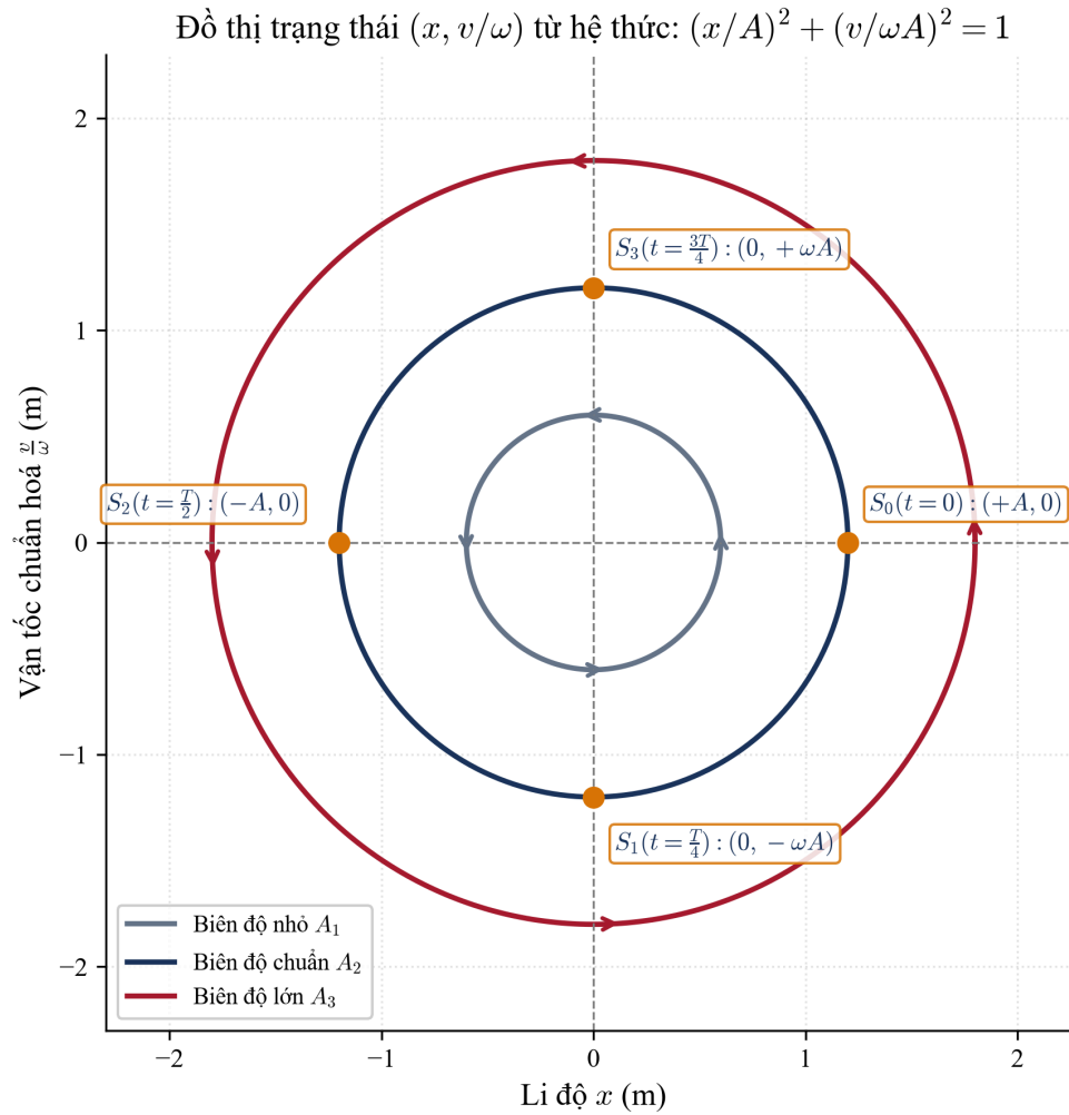
Hình 3: Đồ thị trạng thái (x, v/\omega) biểu diễn quỹ đạo khép kín của dao động điều hòa theo chiều kim đồng hồ.
