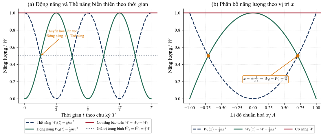
Hình 5: Động năng W_d và Thế năng W_t chuyển hóa tuần hoàn theo thời gian và phân bố theo li độ x .
