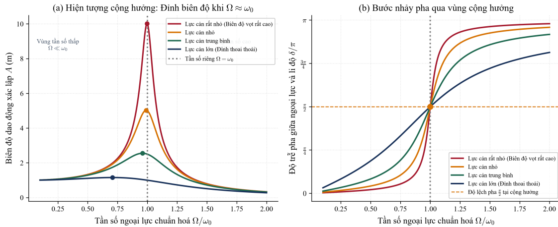
Hình 7: Đường cong cộng hưởng biên độ đạt đỉnh khi tần số ngoại lực trùng khớp với tần số riêng.
