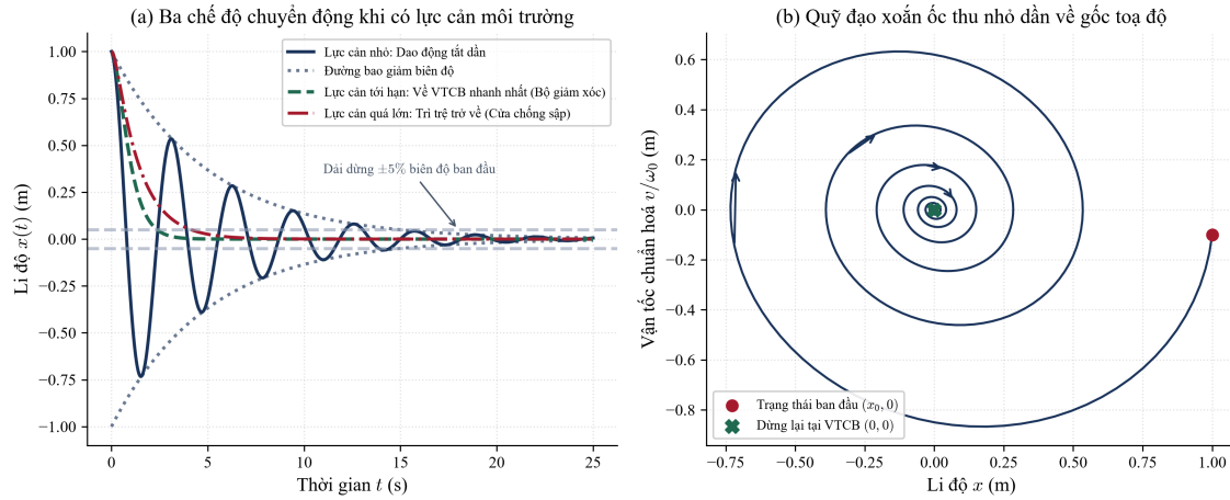
Hình 6: Ba chế độ chuyển động khi có lực cản môi trường và đồ thị trạng thái xoắn ốc.
