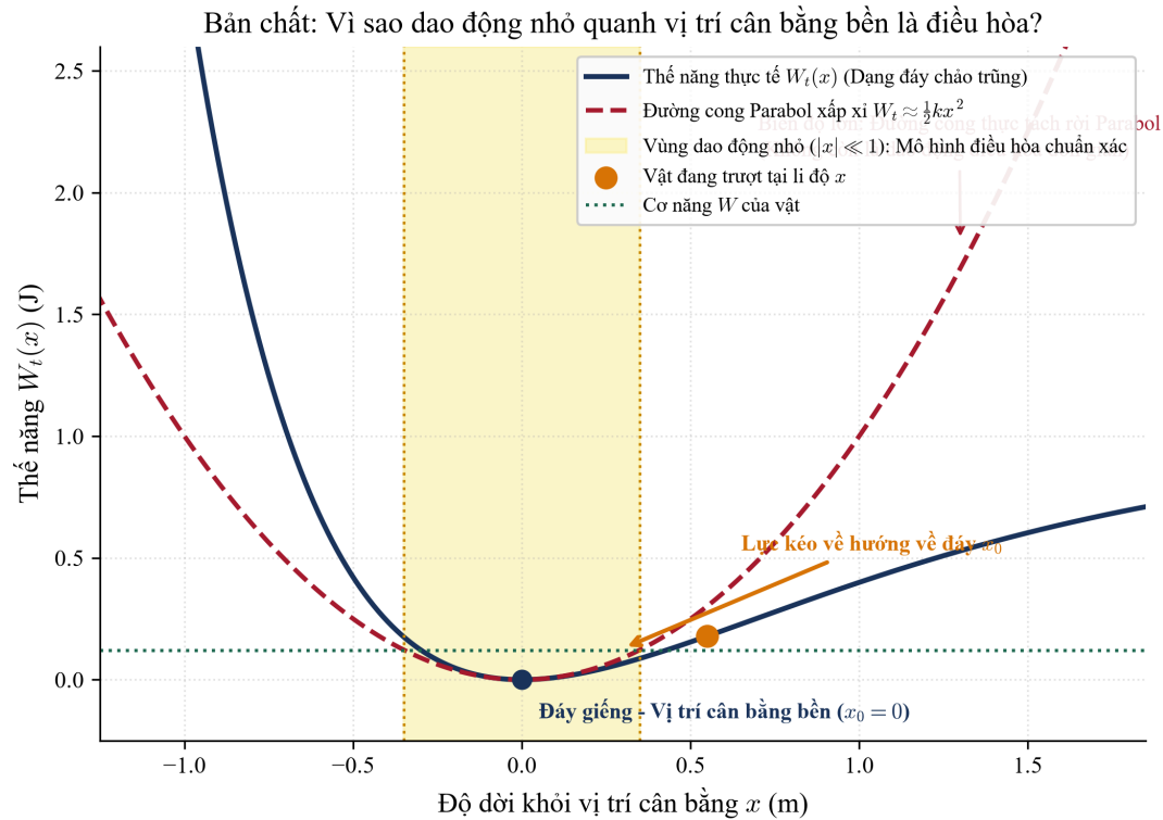
Hình 4: Bản chất hình học của đáy giếng thế năng: Dao động nhỏ quanh vị trí cân bằng bền luôn có thể năng dạng Parabol.
