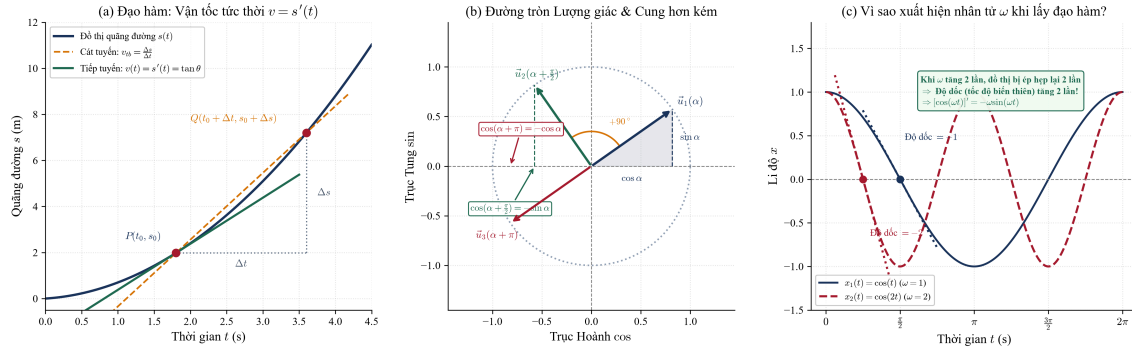
Hình 1: Hình 1.0: Bản chất công cụ Toán học lớp 11: (a) Đạo hàm và vận tốc tức thời, (b) Đường tròn lượng giác giải mã các cung góc, (c) Đạo hàm hàm cosin và nhân tử omega.
