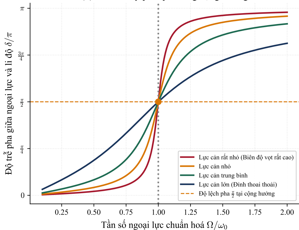
(b) Bước nhảy pha qua vùng cộng hưởng
