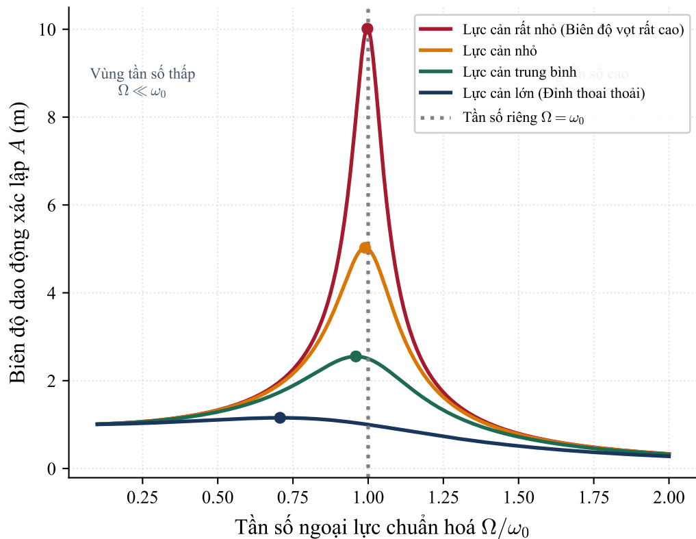
(a) Hiện tượng cộng hưởng: Đỉnh biên độ khi \Omega \approx \omega_0
